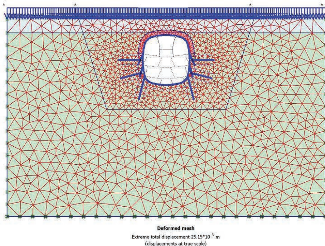
شکل ۱۴: مدل نهایی ساخته شده با مدل رفتاری خاک سخت شونده
