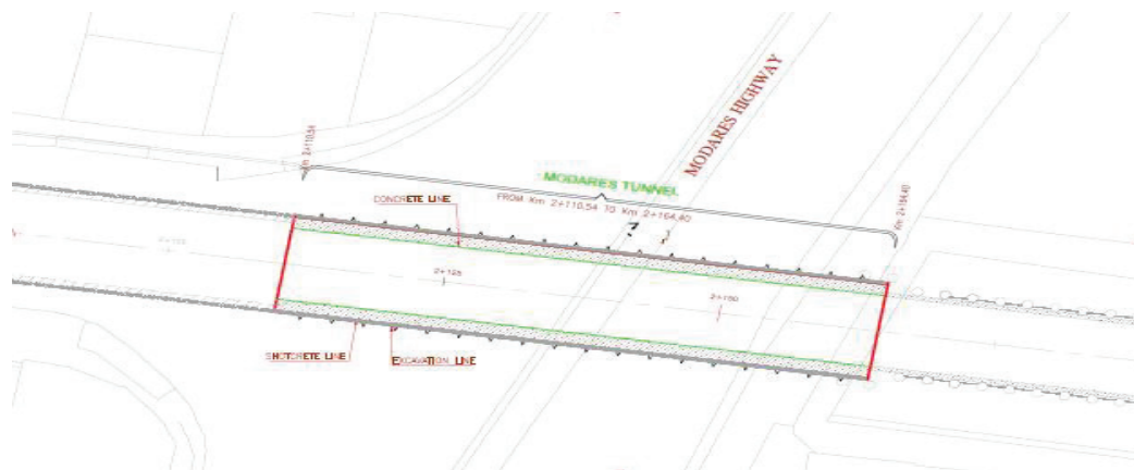
شکل ۷: پلان تونل دوطبقه مدرس [۲۳]
