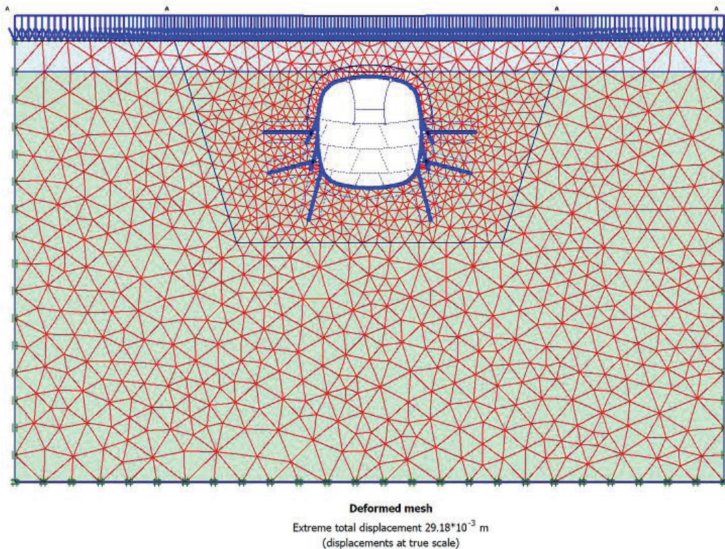
شکل ۱۵: مدل نهایی ساخته شده با مدل رفتاری موهر-کولمب
