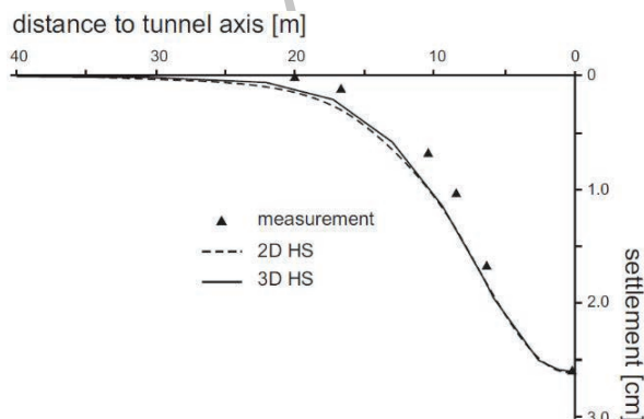
شکل ۵: مقایسه نشست سطح زمین در آنالیز دوبعدی و سه بعدی تونل هین نورد [۸]
