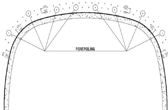
شکل ۱۲: عملیات فورپولینگ تونل مدرس [۲۳]
