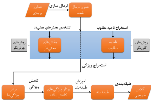
شکل ۱- فلوچارت مراحل کار سیستم‌های کلی‌نگر و جزئی‌نگر.
