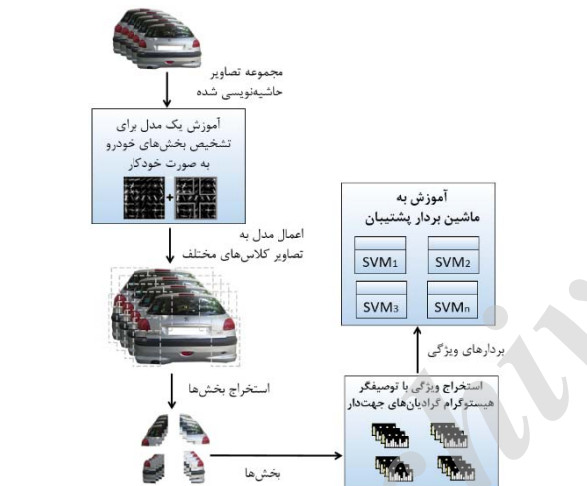
شکل ۱۳ - مراحل آموزش سیستم شناسایی نوع و مدل خودرو با استفاده از استخراج خودکار بخش‌ها
