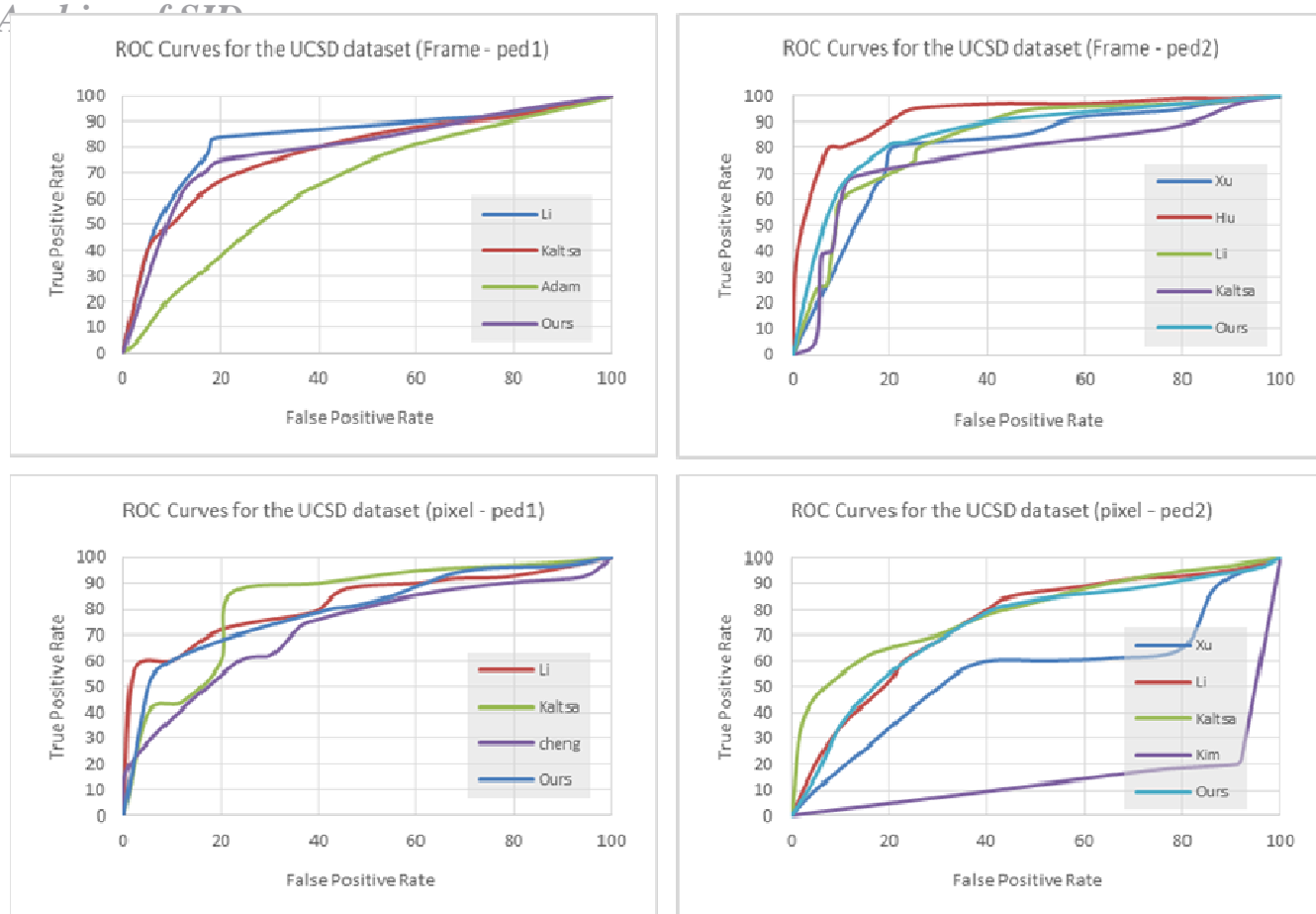
شکل ۸ منحنیهای ROC در مجموعه داده UCSD در سطوح پیکسل و فریم
