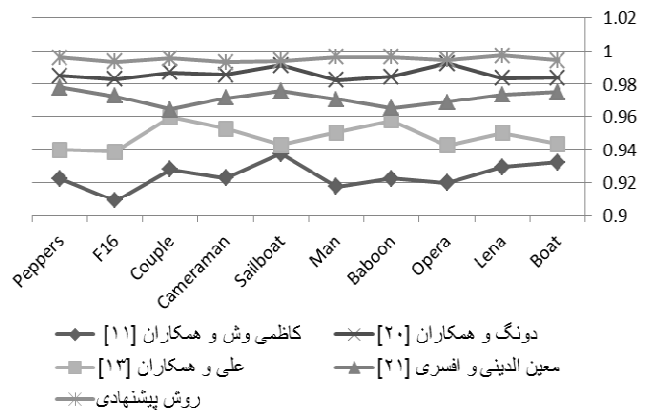
مقادیر SSIM
