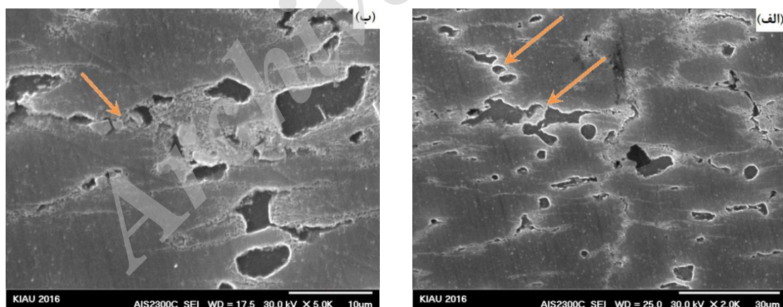
شکل ۹- تصاویر SEM از رسوب‌های شکسته شده در نمونه ریخته‌گری معمولی ۱ پاس ECAP شده در دمای محیط: (الف) رسوب‌های \text{Al}_3\text{Mg}_2 و (ب) رسوب‌های \text{AlFe} .
