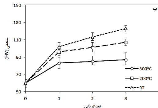
شکل ۶- تاثیر دما و تعداد پاس MDF بر سختی نمونه‌های: (الف) ریختگی معمولی و (ب) ریختگی نیمه‌جامد.
