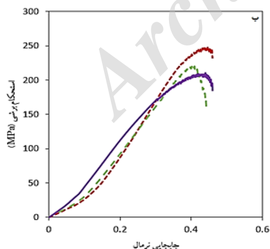
شکل ۷- نمودار تنش برشی - جابجایی نرمال آلیاژ A520 ریختگی معمولی و نیمه‌جامد ECAP و MDF شده در دماهای محیط و 200 و 300 درجه سانتیگراد.
