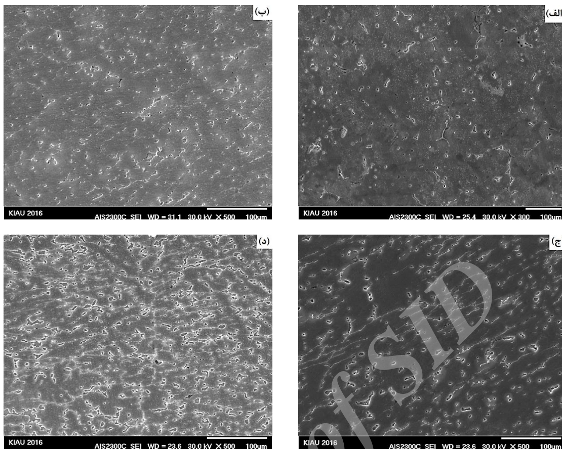
شکل ۸- تصویر SEM، (الف) نمونه نیمه‌جامد ۳ پاس ECAP شده در دمای محیط، (ب) نمونه نیمه‌جامد ۳ پاس ECAP شده در دمای 200^{\circ}\text{C} و (ج) نمونه نیمه‌جامد ۳ پاس ECAP شده در دمای 300^{\circ}\text{C} و (د) نمونه ریخته‌گری معمولی ۱ پاس ECAP شده در دمای محیط.
