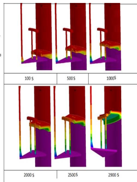
شکل ۳- نتایج شبیه‌سازی توزیع حرارت در میله GTD111-DS در مقطع برش شکل (۲-ج)
