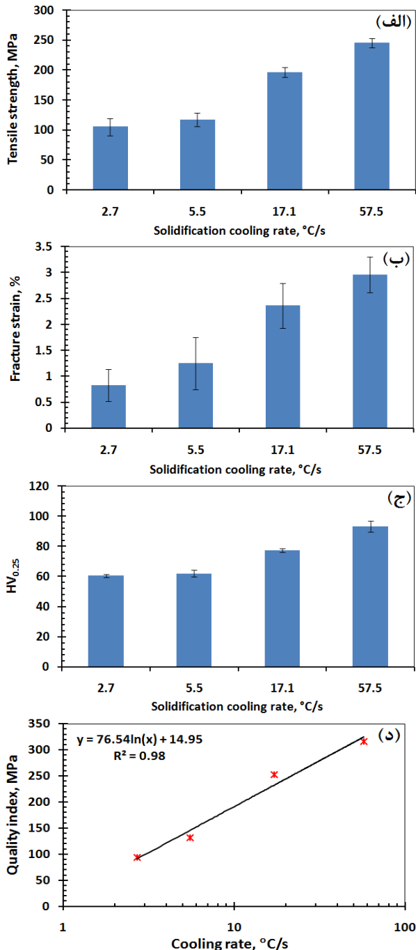
شکل ۵- تاثیر سرعت انجماد بر (الف) استحکام کششی، (ب) درصد ازدیاد طول، (ج) سختی میکروسکوپی فاز آلفا (زمینه)، (د) اندیس کیفیت کامپوزیت Al-15Mg_2Si
