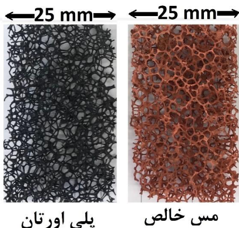
شکل ۱- نمایی از تبدیل اسفنج پولی اورتان به فوم مسی [۵، ۹].
