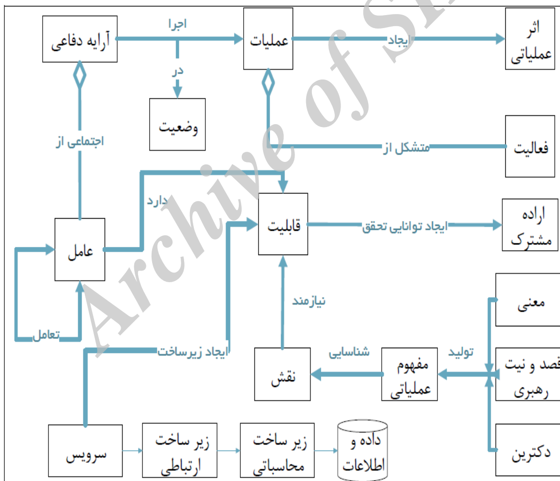
شکل ۹. فرامدل جامع برنامه‌ریزی قابلیت آرایه‌های دفاعی
