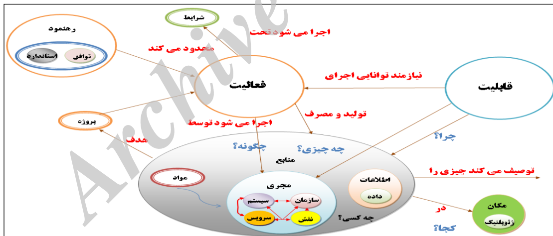
شکل ۳. قابلیت و مفاهیم مرتبط در چارچوب معماری دودف (USDOD, 2010)
