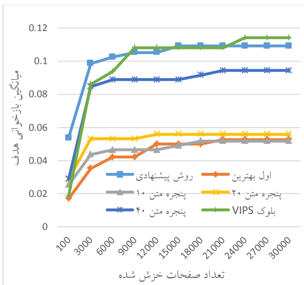
شکل ۱۳. میانگین بازخوانی هدف روش‌ها برای موضوعات مختلف
