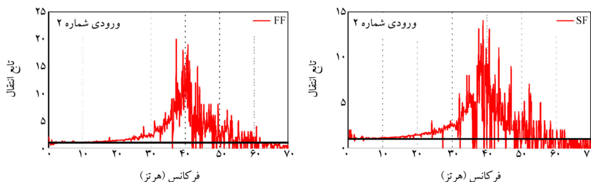
شکل (8): تابع تبدیل شتاب مدل‌های SF و FF برای تحریک‌های ورودی مختلف در مقیاس مدل
