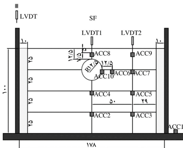
شکل (6): ابزارگذاری مدل SF (ابعاد بر حسب سانتی‌متر و در مقیاس مدل می‌باشد)
