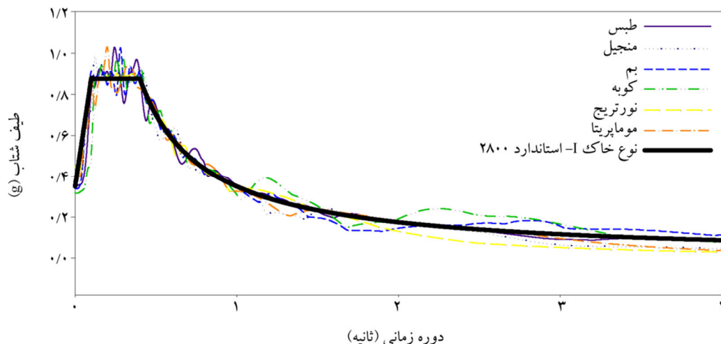
شکل (15): طیف پاسخ شتاب زلزله‌های انتخاب شده در مطالعه پارامتری سازگار شده با طیف استاندارد 2800 برای زمین نوع 1
