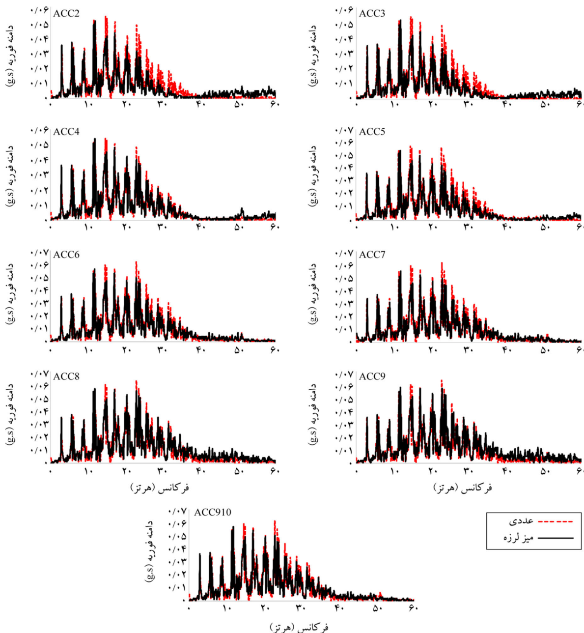
شکل (11): مقایسه طیف فوریه شتاب در موقعیت‌های مختلف در مدل عددی و آزمایشگاهی FF تحت تحریک ورودی شماره 2
