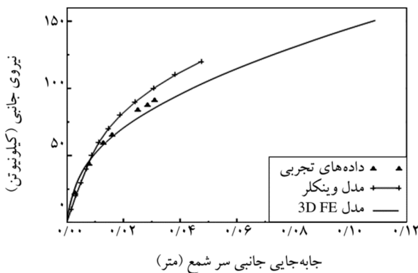
شکل (4): مقایسه‌ی نتایج تحلیل استاتیکی مدل اجزاء محدود با نتایج آزمایشگاهی و روش وینکلر
