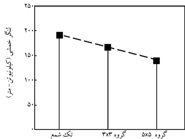
شکل (10): مقایسه‌ی لنگر خمشی بیشینه در فصل مشترک دو لایه برای شمع منفرد و شمع مرکزی در گروه‌های 5×5 و 3×3
