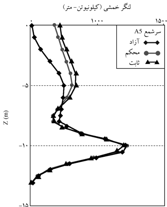
شکل (11): مقایسه‌ی پوش لنگر خمشی شمع A-5 به قطر D = 0.9m در گروه شمع 5×5 برای شرایط گیرداری متفاوت
