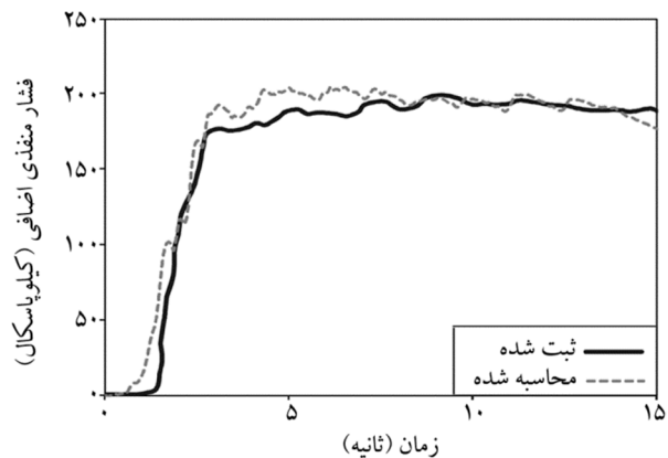
شکل (11): تاریخچه فشار آب منفذی اضافی در روش عددی ( R=8 ) و آزمایشگاهی برای عمق 20 متر
