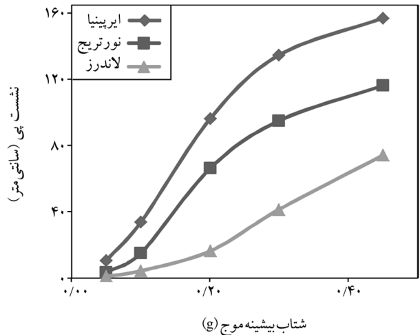
شکل (14): مقادیر نشست سازه برای موج‌های ورودی مختلف بر حسب شتاب بیشینه موج ورودی
