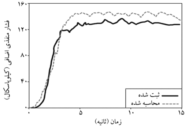
شکل (10): تاریخچه فشار آب منفذی اضافی در روش عددی ( R=8 ) و آزمایشگاهی برای عمق 12 متر
