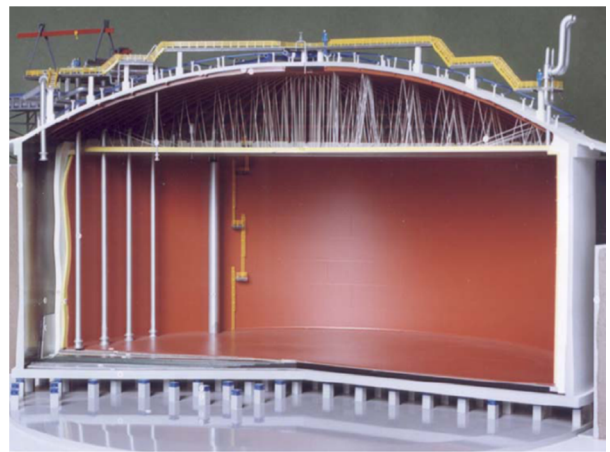
شکل (1): نمای کلی مخازن ذخیره‌ی گاز طبیعی اجرا شده در یونان (Revithoussa LNG Terminal) و محافظت‌شده با جداسازهای لرزه‌ای
