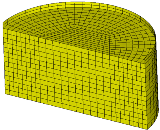
شکل (2): شبکه‌بندی مدل اجزای محدود مورد استفاده برای مخازن مجهز به جداساز لرزه‌ای
