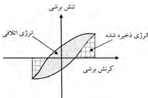
شکل (8): نمای شماتیک یک حلقه هیستریزس در صفحه تنش-کرنش
