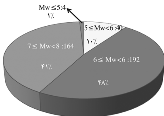
شکل (7): تقسیم‌بندی حرکات زلزله‌ها بر اساس بزرگای لرزه‌ای
