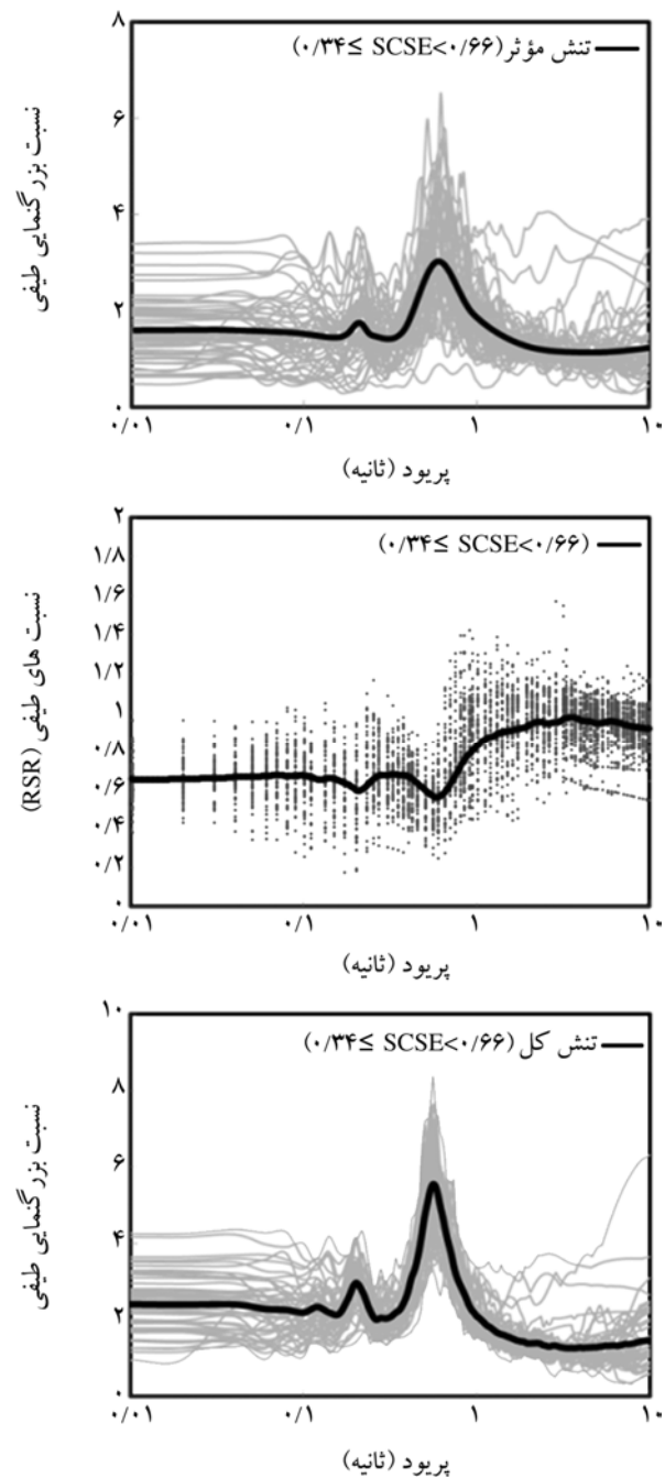
شکل 13): میانگین الگوهای بزرگنمایی و نسبت طیف‌های پاسخ در دو تحلیل تنش کل و تنش مؤثر در محدوده‌های متوسط ( 0/34 \leq SCSE < 0/66 )
