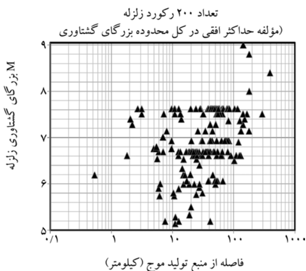
شکل (6): نمایش بزرگای زلزله به همراه فاصله از منبع تولید آن
