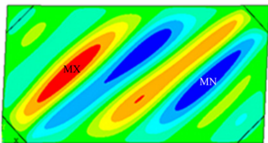
شکل (الف) با سخت‌کننده
