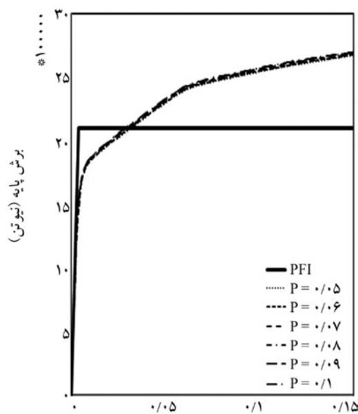
تغییر مکان (متر) (پ) ضخامت ورق ۰/۰۰۷ متر
