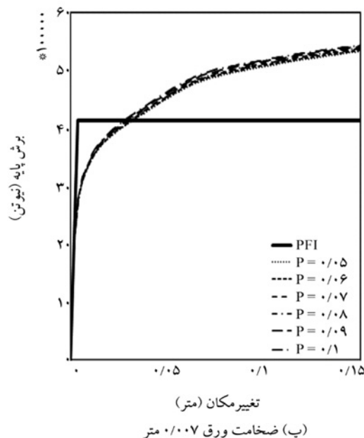
شکل (۷): منحنی بار تغییر مکان دیوار برشی فولادی مستطیل شکل به همراه منحنی PFI
