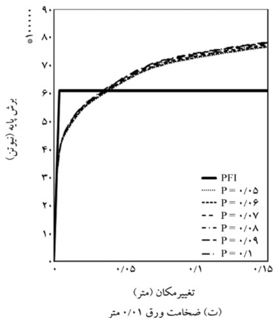
شکل (۷): منحنی بار تغییر مکان دیوار برشی فولادی مستطیل شکل به همراه منحنی PFI
