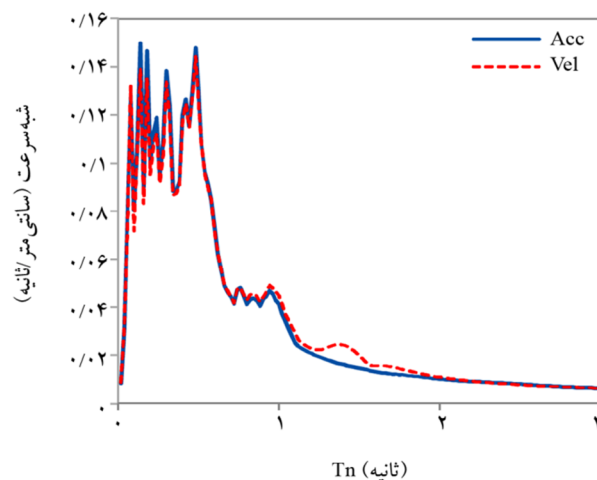
(پ) رکورد شماره ۴ در راستای غربی - شرقی
