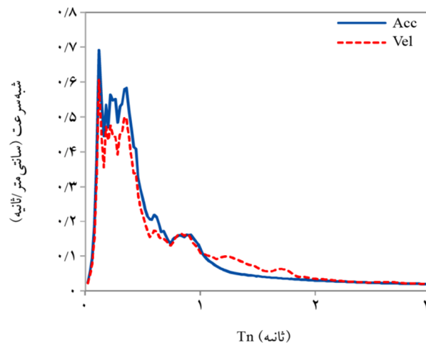
(الف) رکورد شماره ۱ در راستای شمالی - جنوبی
