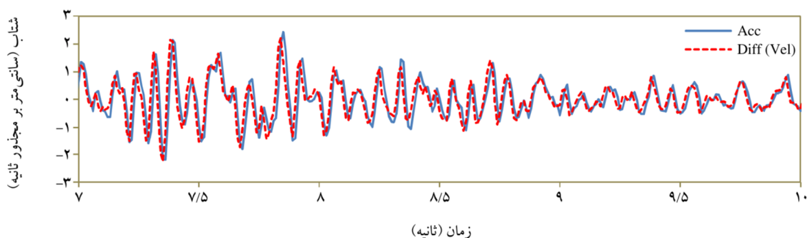
(ت) رکورد شماره ۴ در راستای قائم
