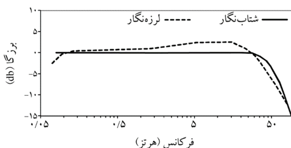
شکل (۲): پاسخ دستگاهی شتاب‌نگار و لرزه‌نگار مورد استفاده
