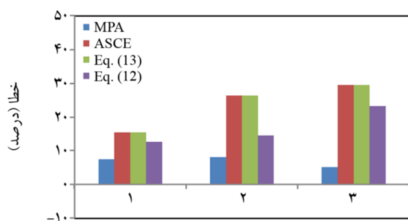
شماره قاب ساختمانی (ب) زلزله‌های دور به گسل
