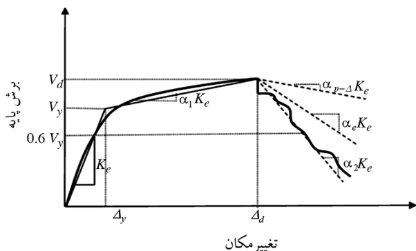
شکل (۱): منحنی‌های نیرو-تغییر مکان ایده‌آل [۵]
