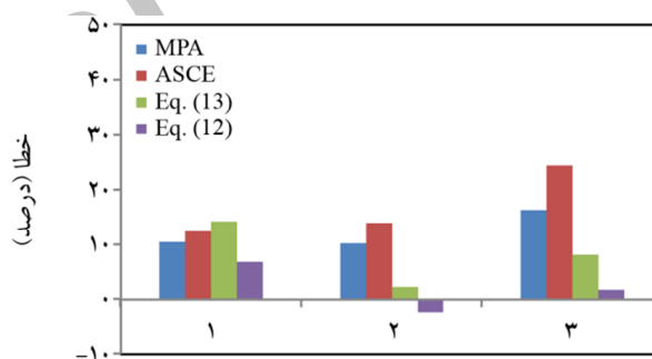
شماره قاب ساختمانی (الف) زلزله‌های نزدیک به گسل
