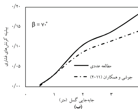
شکل (۵): تغییرات بیشینه کرنش‌های فشاری ایجاد شده در لوله برای زاویه شیب الف) ۴۰ درجه و ب) ۷۰ درجه.
