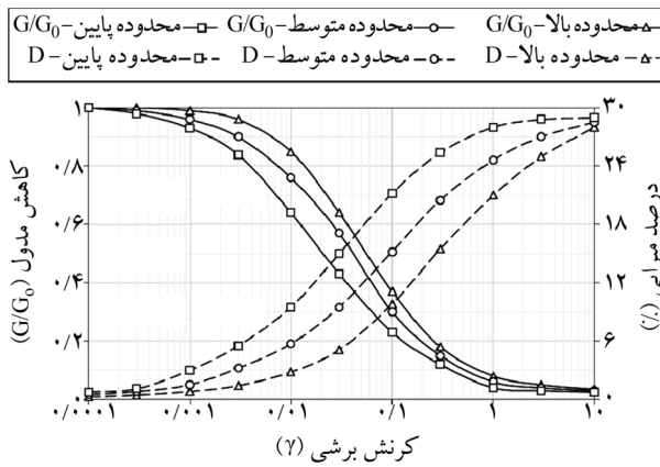
شکل (۵): تغییرات مدول برشی و میرایی در مقابل کرنش برشی برای ماسه [۲۶].
