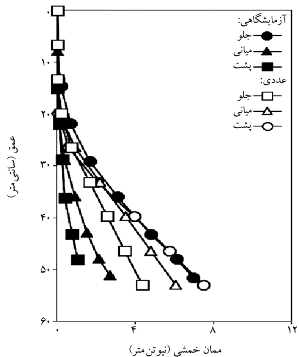
شکل (۱۵): پروفیل تغییرات ممان خمشی شمع‌های ستون میانی در مدل آزمایشگاهی و عددی.
