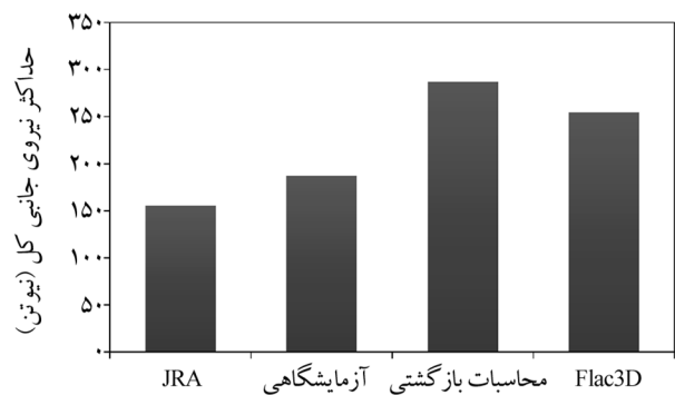
شکل (۱۷): حداکثر نیروی جانبی کل وارد بر گروه شمع در روش‌های مختلف.
