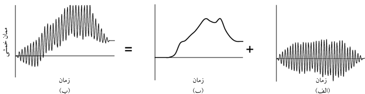
شکل (۱۳): تجزیه نمونه‌ای از یافته‌های ثبت شده ممان: (الف) مؤلفه یک‌سویه؛ (ب) مؤلفه چرخه‌ای؛ (پ) یافته‌های ثبت شده.
