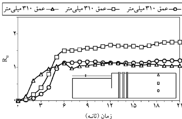
شکل (۸): تاریخچه زمانی نسبت اضافه فشار آب حفره‌ای در اعماق مختلف دور از گروه شمع در مدل عددی.
