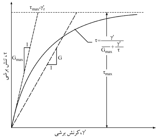
شکل (۴): منحنی‌های بیرونیکی [۲۵].
