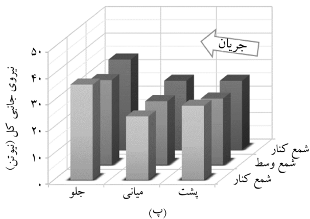
شکل (۱۶): توزیع حداکثر نیروی جانبی کل در گروه شمع: (الف) مدل آزمایشگاهی؛ (ب) روش محاسبات بازگشتی؛ (پ) مستخرج از برنامه FLAC3D.
