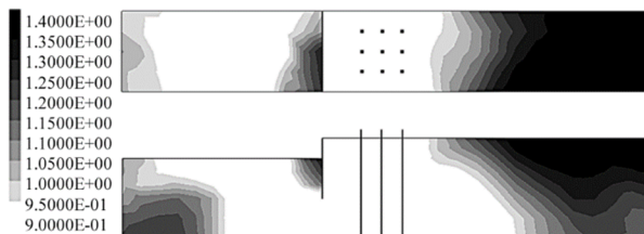
شکل (۹): پلان و مقطع حداکثر نسبت اضافه فشار آب حفرةای R_{II} .
