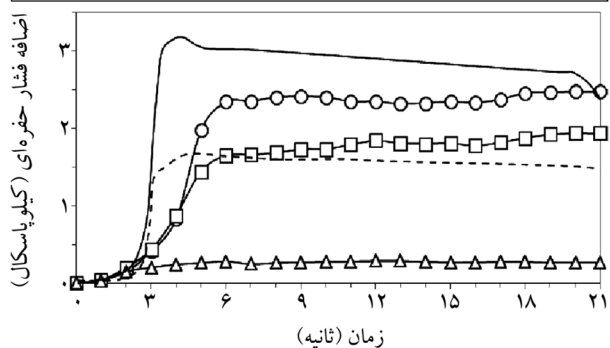
شکل (۶): تاریخچه زمانی فشار آب حفره‌ای در اعماق مختلف دور از گروه شمع.
