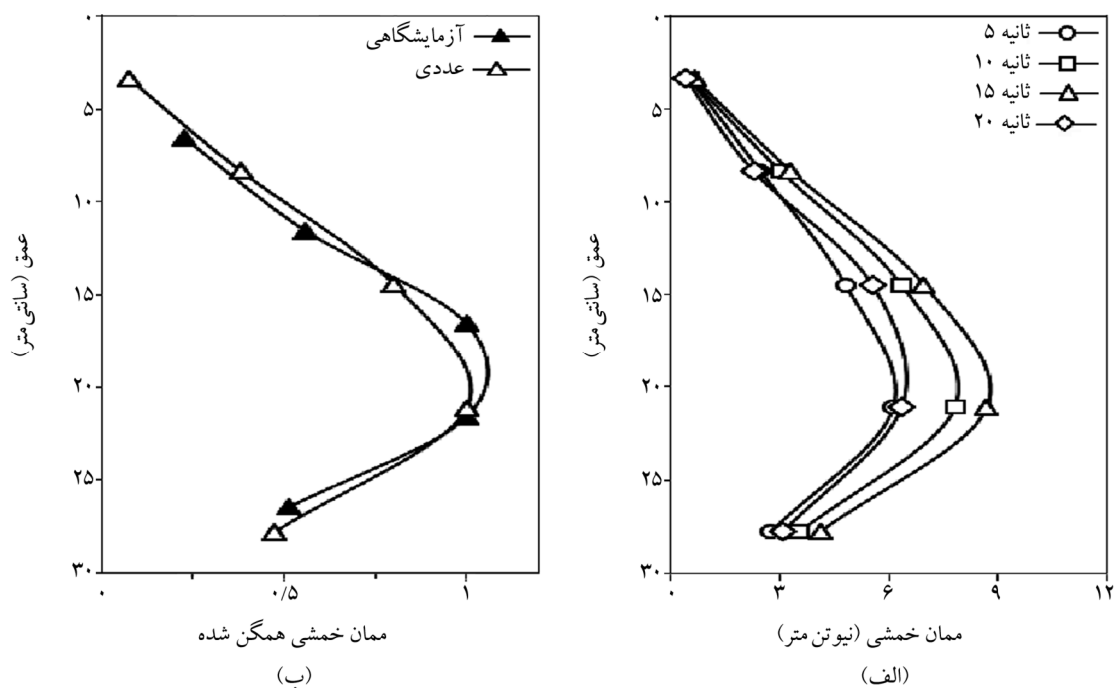
شکل (۱۸): پروفیل ممان خمشی دیوار: (الف) در زمان‌های مختلف برای مدل عددی؛ (ب) همگن شده برای مدل آزمایشگاهی با فرکانس ۱۰ هرتز و دامنه Gal ۳۰۰ و مدل عددی با فرکانس ۵ هرتز و دامنه Gal ۱۵۰.
