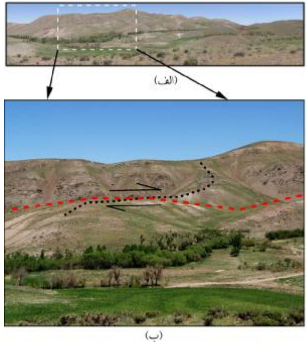
شکل (۱۱): الف) نمای دور از مورفولوژی، ب) تصویری از یک پشته جابه‌جا شده که حرکت راست‌بر گسله کوشک نصرت را نشان می‌دهد (روستای بند امیر).
