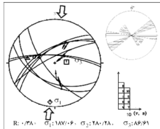
شکل (۶): محاسبه سازوکارهای کانونی به روش برگشتی. بالای تصویر سمت راست نمودار گل سرخی، پایین سمت راست نمودار زاویه ناهمخوانی و سمت چپ تانسور تنش حل شده با نمایش سازوکارها. پایین تصویر مقدار بیضوی تنش (R) و مقادیر تنش‌های پیشینه تا کمینه دیده می‌شود.
