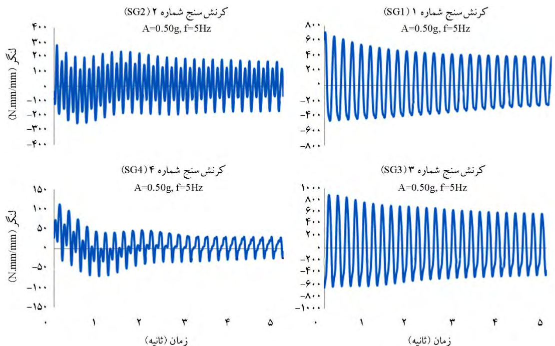
شکل (۱۶): نمودارهای تاریخچه زمانی لنگر ثبت شده در نقاط مختلف مدل تونل برای A=0.50g و f=5Hz .
