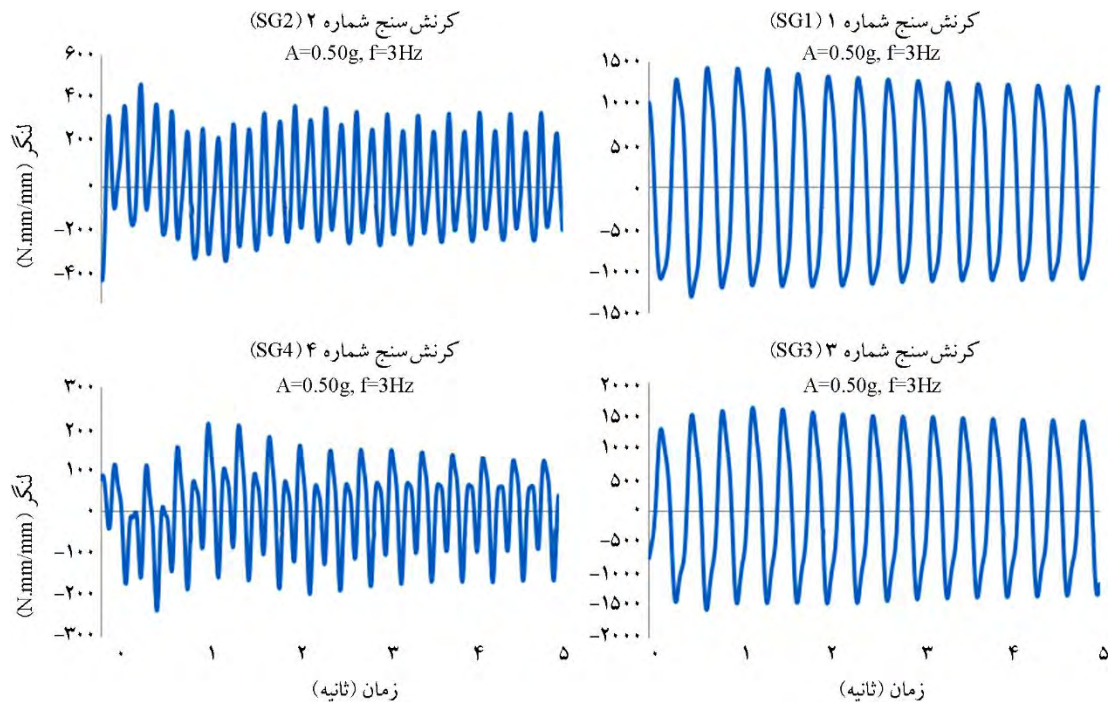
شکل (۱۵): نمودارهای تاریخچه زمانی لنگر ثبت شده در نقاط مختلف مدل تونل برای A=0.50g و f=3Hz .
