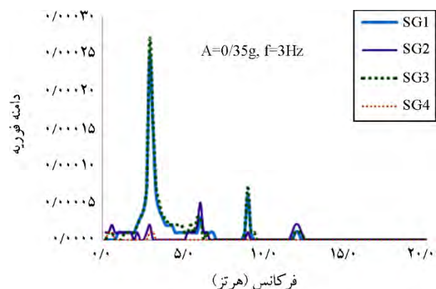
شکل (۲۰): منحنی پاسخ کرنش‌های خمشی (SG1، SG2، SG3 و SG4) برای A=0.35g و f=3Hz
