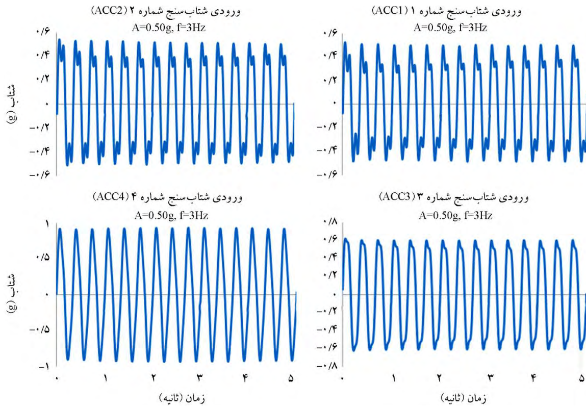
شکل (۱۰): نمودارهای تاریخچه زمانی شتاب ثبت شده برای A=0.50g و f=3Hz .
