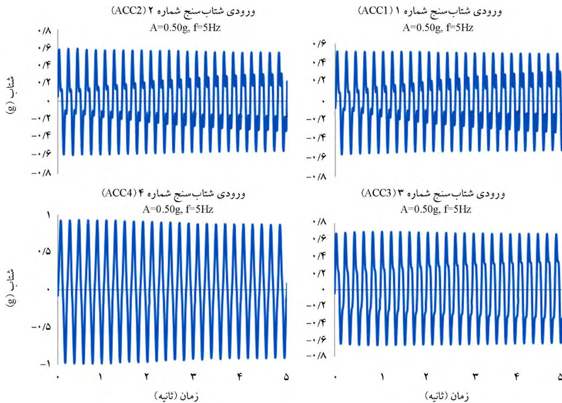
شکل (۱۱): نمودارهای تاریخچه زمانی شتاب ثبت شده برای A=0.50g و f=5Hz .
