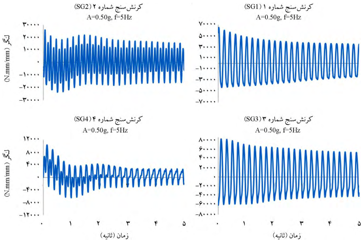
شکل (۱۸): نمودارهای تاریخچه زمانی لنگر در نمونه اصلی در محل کرنش سنج‌های SG1، SG2، SG3 و SG4 برای A=0.50g و f=5Hz .
