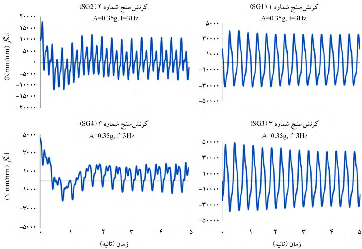
شکل (۱۷): نمودارهای تاریخچه زمانی لنگر در نمونه اصلی در محل کرنش سنج‌های SG1، SG2، SG3 و SG4 برای A=0.35g و f=3Hz .
