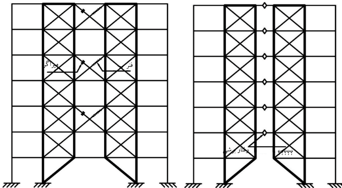
شکل (۳): دو دهانه مهاربندی به عنوان هسته صلب با تکیه گاه مفصل در کنار و تیر پیوند با رفتار برشی در برخی از طبقات (سمت راست); دو دهانه مهاربندی به عنوان هسته صلب با تکیه گاه مفصل در کنار و فنر پیش فشرده و میراگر لزوج در برخی از طبقات (سمت چپ).
