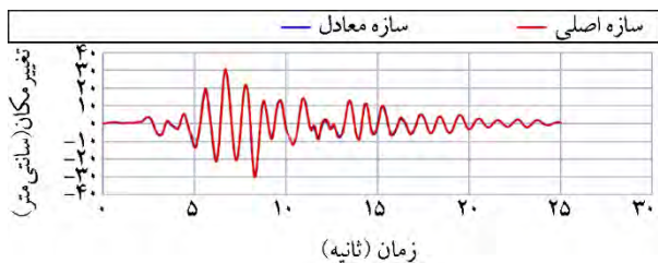
شکل (۱۰): منحنی تغییر مکان ارتجاعي سازه‌ی معادل و سازه اصلی برای زلزله مصنوعی شماره ۴ با نصف شتاب ثقل.
