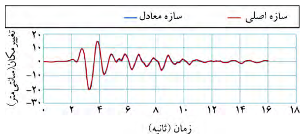
شکل (۸): منحنی تغییر مکان ارتجاعي سازه‌ی معادل و سازه اصلی برای زلزله بم با نصف شتاب ثقل.
