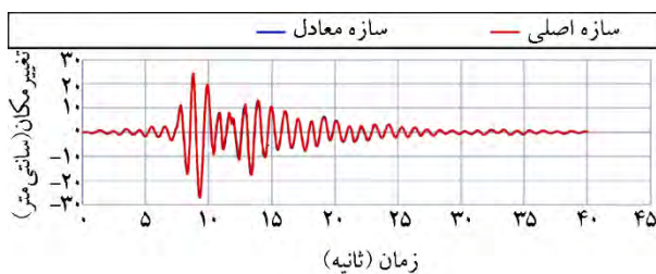
شکل (۹): منحنی تغییر مکان ارتجاعي سازه‌ی معادل و سازه اصلی برای زلزله کوبه با نصف شتاب ثقل.
