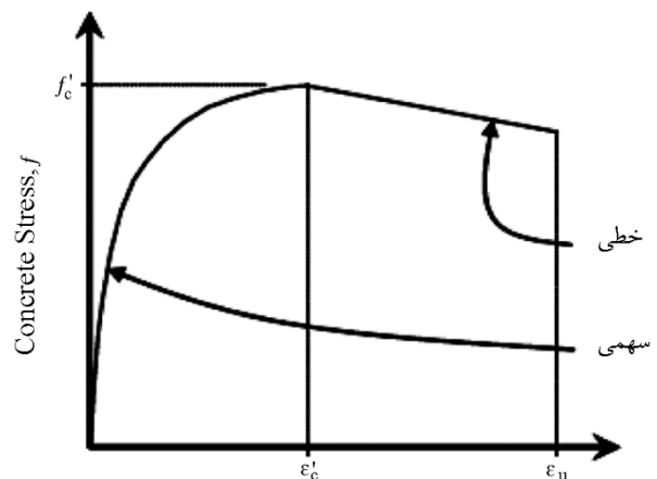
شکل (۳): قسمت فشاری منحنی رفتاری بتن ساده.
