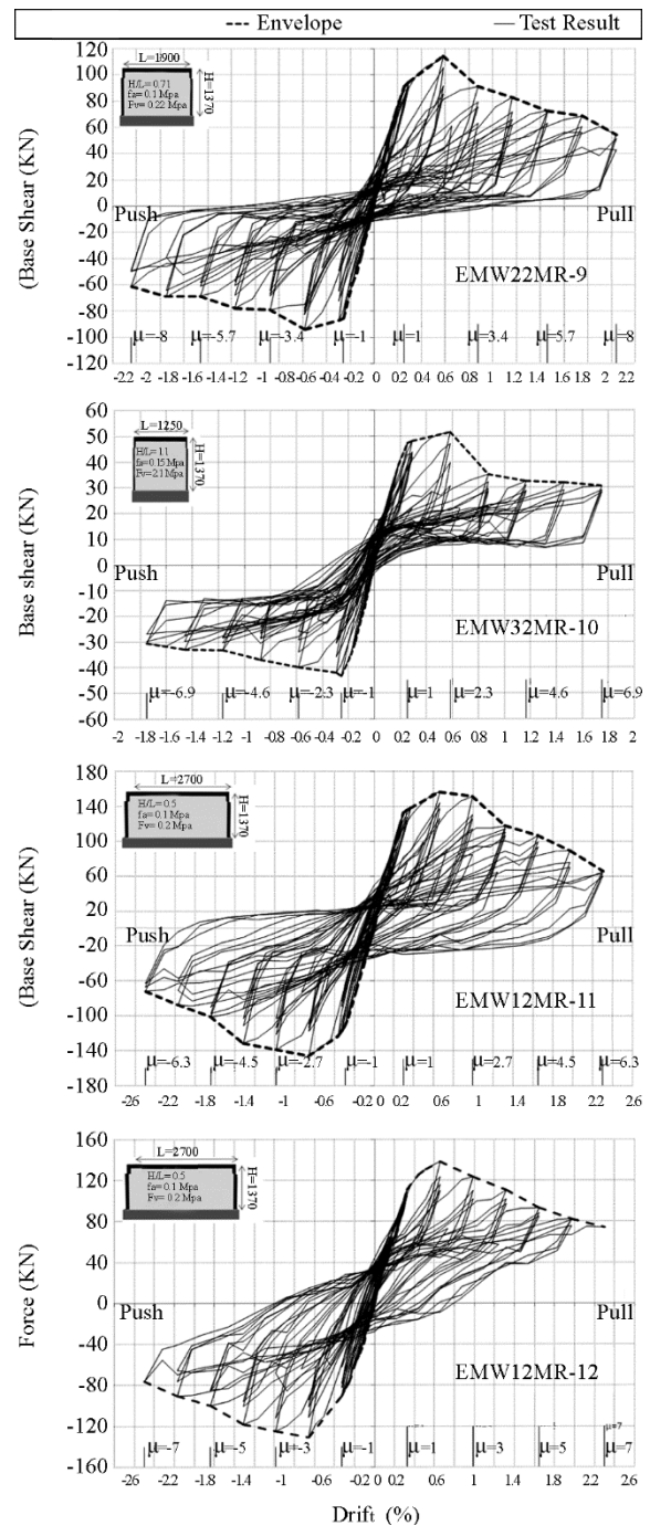
شکل (۸): رفتار چرخه‌ای نمونه‌های آزمایشگاهی [۲۳].
