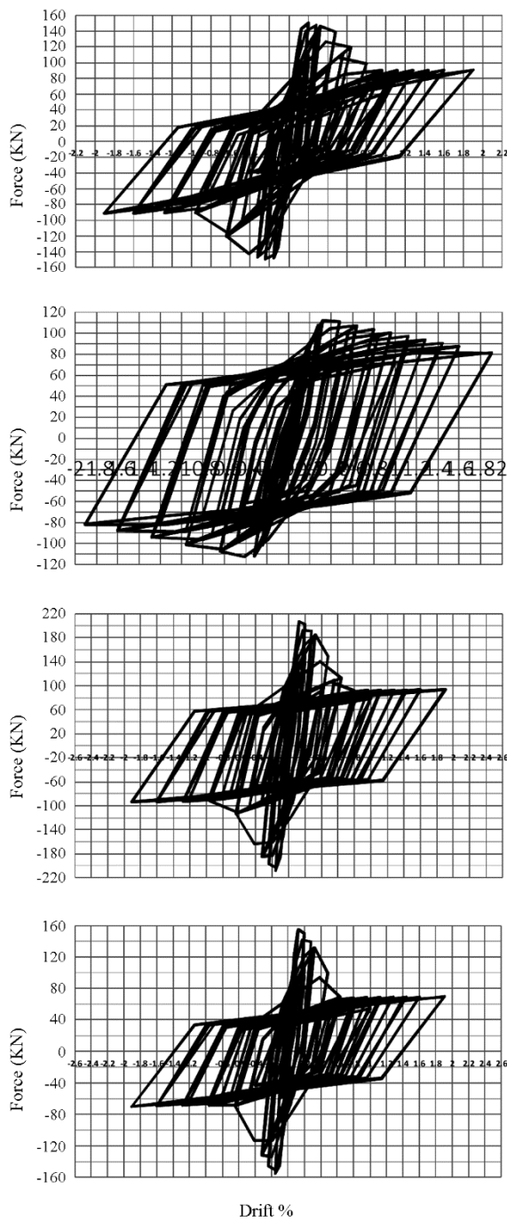
شکل (۹): نتایج تحلیلی رفتار چرخه‌ای.
