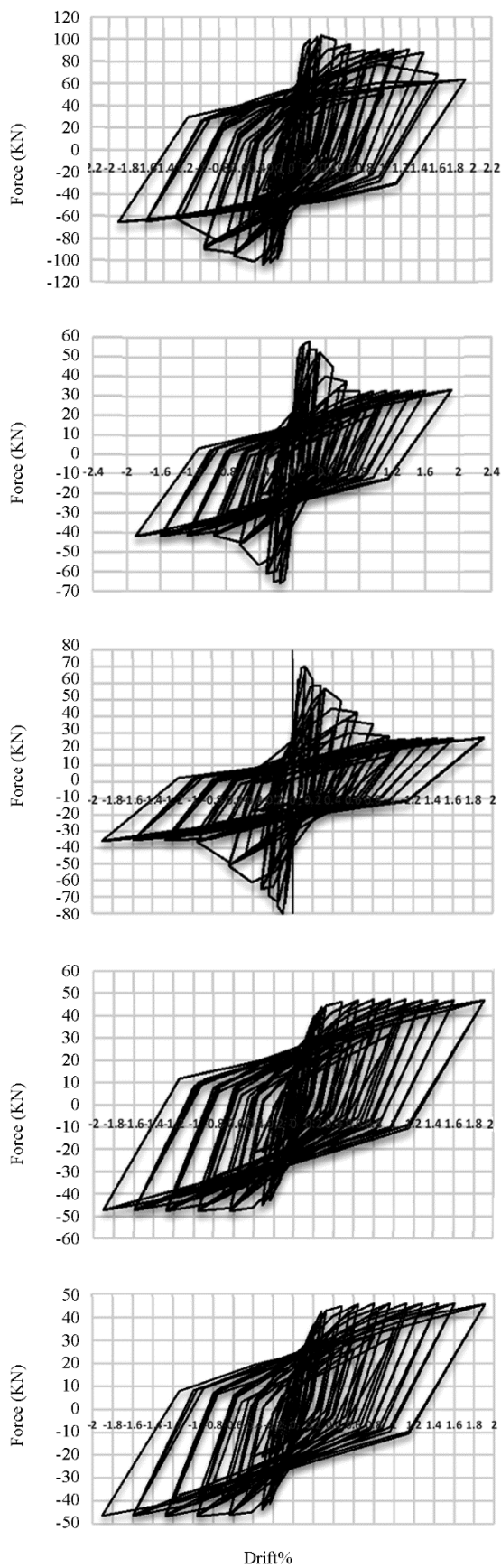
شکل (۷): نتایج تحلیلی رفتار چرخه‌ای.
