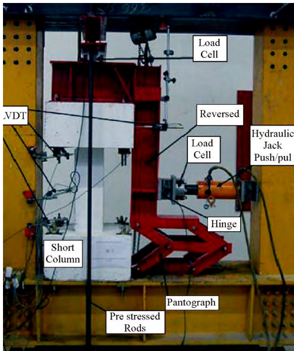
شکل (۳): دستگاه آزمایش ستون های کوتاه بتن مسلح [۷].
