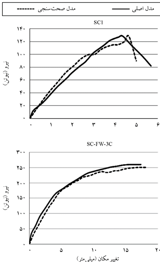
شکل (۴): مقایسه مدل نرم‌افزاری و آزمایشگاهی نمونه‌های SC1 و SC-FW-3C.
