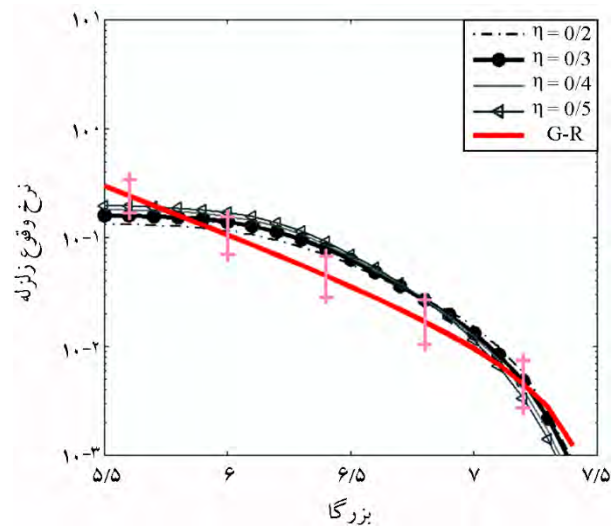
شکل (۴): نمودار تکرار- بزرگای به دست آمده به ازای مقادیر مختلف \eta در مقایسه با رابطه تجربی. مقادیر انحراف معیار رابطه تجربی به صورت خطوط قائم نشان داده شده است.
