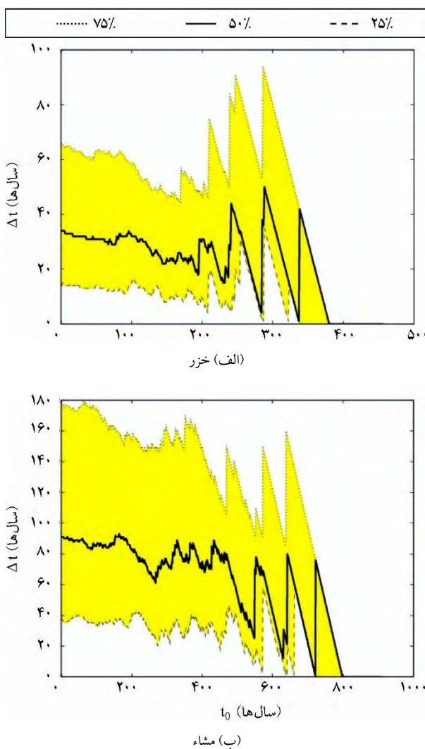
شکل (۹): توزیع زمان مورد انتظار (EWT) برای وقوع زلزله با بزرگای بیشتر از ۶ در گسل (الف) خزر، (ب) مشاء برای احتمالات ۲۵، ۵۰ و ۷۵ درصد.
