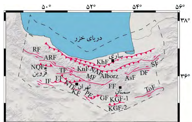
شکل (۱): نقشه گسل‌های فعال در ناحیه البرز (خط چین بیانگر محدوده ناحیه مورد مطالعه می‌باشد). RF: رودبار، ARF: الموترود، TF: طالقان، NQF: شمال قزوین، EF: اشتهارد، IF: ایپک، FF: فیروزکوه، NAF: شمال البرز، GF: گرمسار، KGF-1: کوه گچاب-۱، KGF-2: کوه گچاب-۲، MF: مشاء، TOF: تروند، PF: پیشوا، DF: دامغان، NTF: شمال تهران، ASF: آستانه، KhF: خزر، KnF: کندوان، KF: کهریزک، SF: شاور
