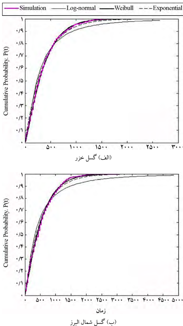
شکل (۶): تابع توزیع تجمعی دوره بازگشت زلزله‌ها +M6.
