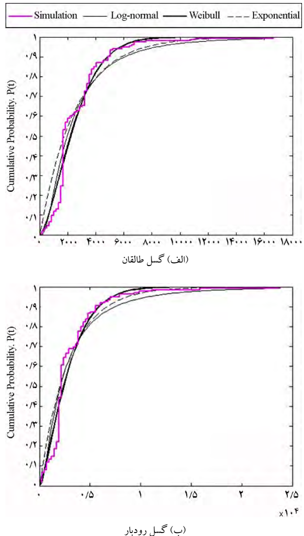
شکل (۷): تابع توزیع تجمعی دوره بازگشت زلزله‌ها M6+ .
