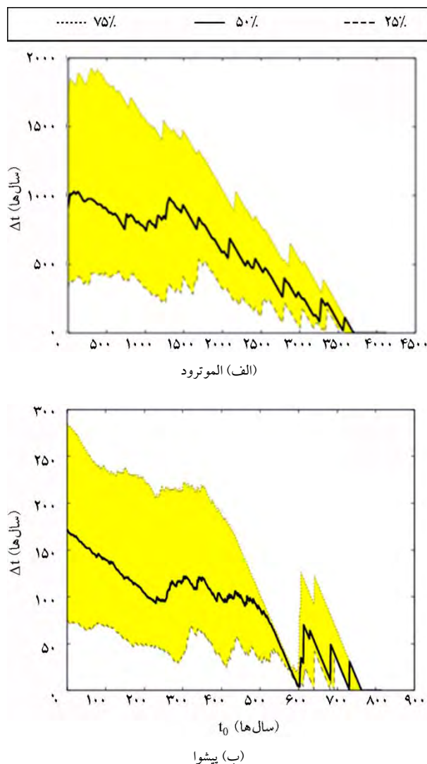
شکل (۸): توزیع زمان مورد انتظار (EWT) برای وقوع زلزله با بزرگای بیشتر از ۶ در گسل (الف) الموترود و (ب) پیشوا برای احتمالات ۲۵، ۵۰ و ۷۵ درصد.
