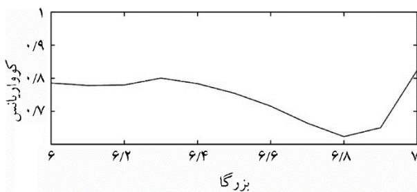
شکل (۵): تغییرات انحراف معیار دوره بازگشت زلزله‌ها در گسل شمال تهران.
