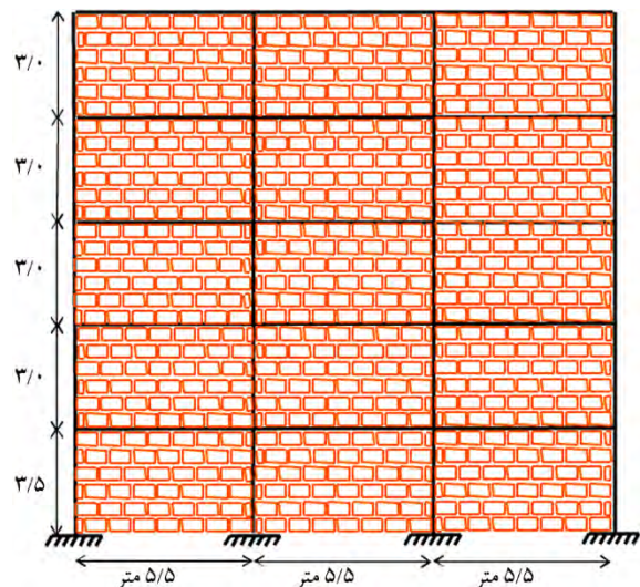
شکل (۱۳): قاب مورد بررسی.
