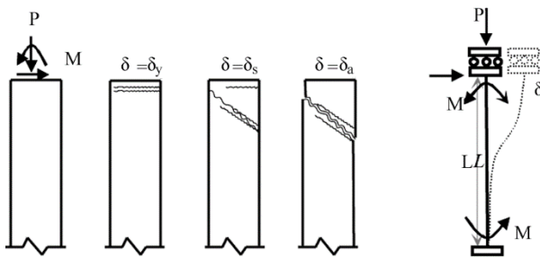
شکل (۸): تغییر شکل انحنا مضاعف ستون‌ها.
