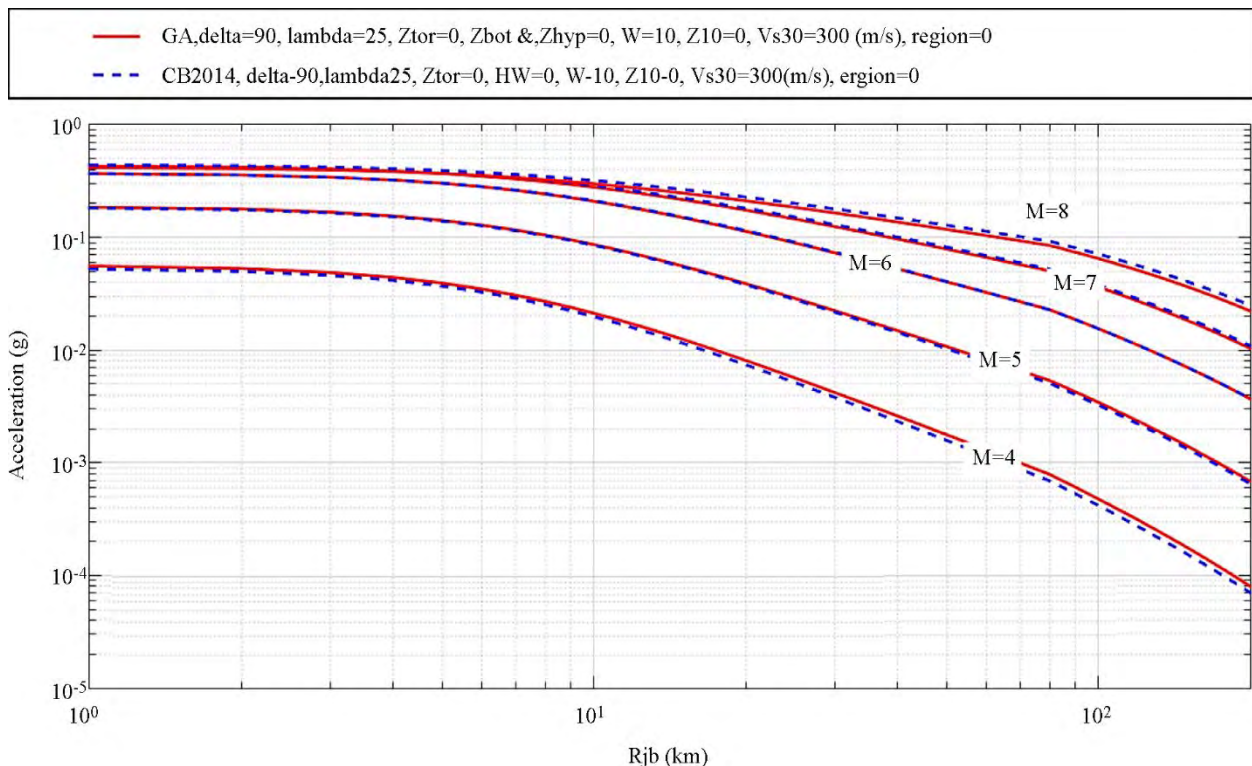
شکل (۱۱): مقایسه PGA رابطه ارائه شده با رابطه CB 2014 در برابر پارامتر بزرگا. (Zbot & Zhyp=0, Fhw=0, W=10, Z10=0, Vs30=300(m/s), region=0, delta=90, lambda=25, Ztor=0)
