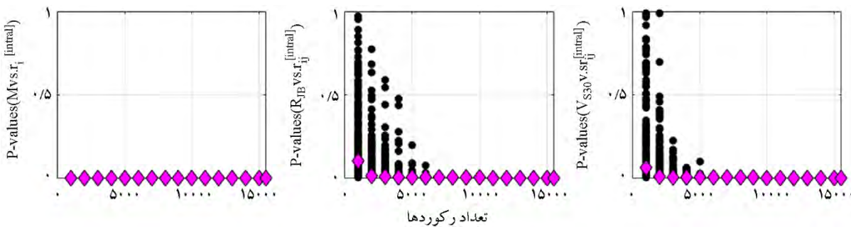
شکل (۸): تحلیل حساسیت مدل آبراهامسون و سیلوا ۲۰۱۴ [۱۴] بر اساس مجموعه داده‌های NGA شامل ۱۵۴۹۳ شتاب‌نگاشت.
