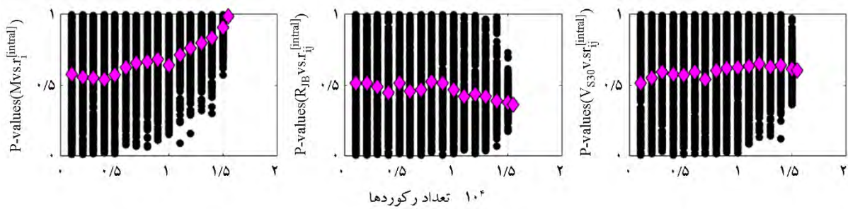
شکل (۷): تحلیل حساسیت مدل آبراهامسون و سیلوا ۲۰۱۴ بهینه شده بر اساس مجموعه داده‌های NGA شامل ۱۵۴۹۳ شتاب‌نگاشت.
