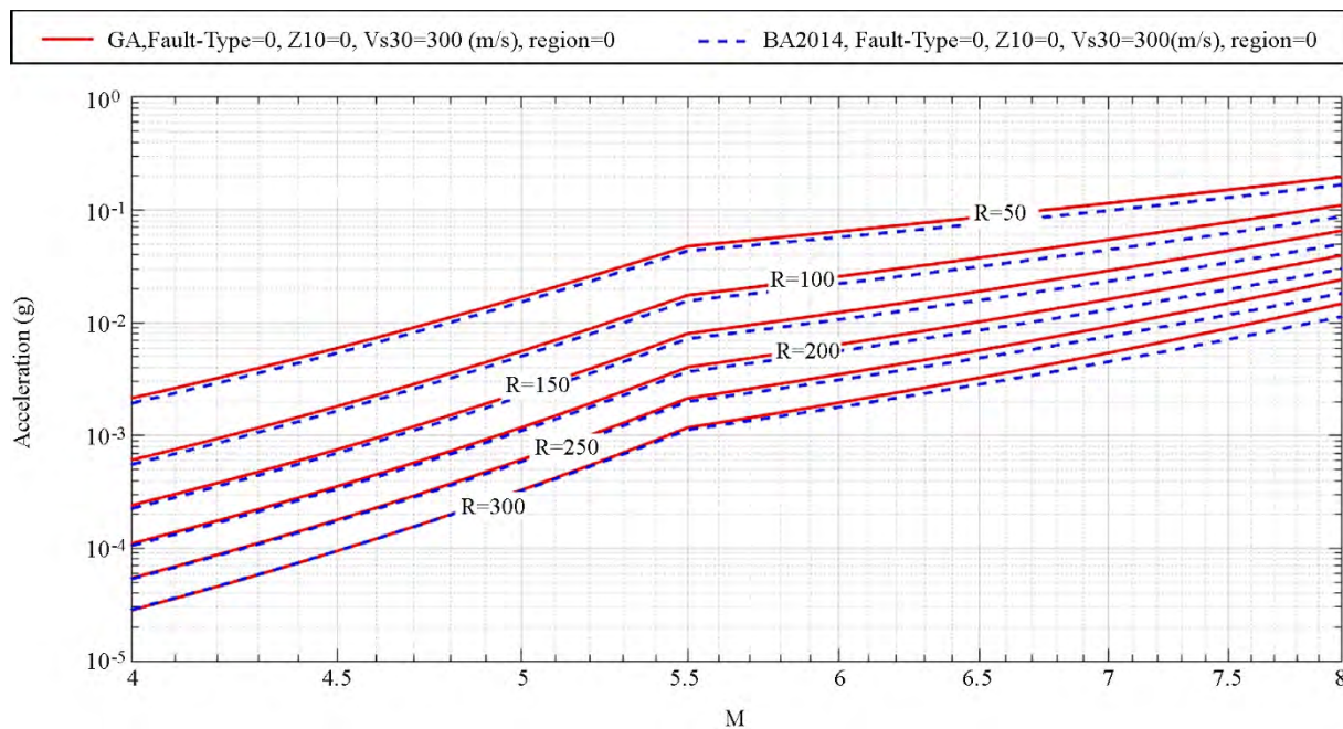
شکل (۱۶): مقایسه رابطه ارنانه شده با رابطه BA 2014 در برابر پارامتر فاصله (Fault-Type=0, Z10=0, Vs30=300(m/s), region=0).
