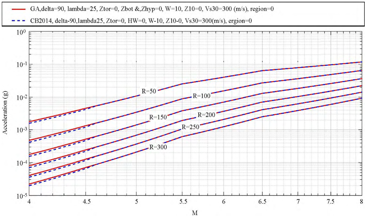
شکل (۱۲): مقایسه PGA رابطه ارائه شده با رابطه CB 2014 در برابر پارامتر فاصله. ( \Delta=90, \lambda=25, Z_{tor}=0, Z_{bot} \& Z_{hyp}=0, F_{hw}=0, W=10, Z_{10}=0, V_s=300(m/s), region=0 )
