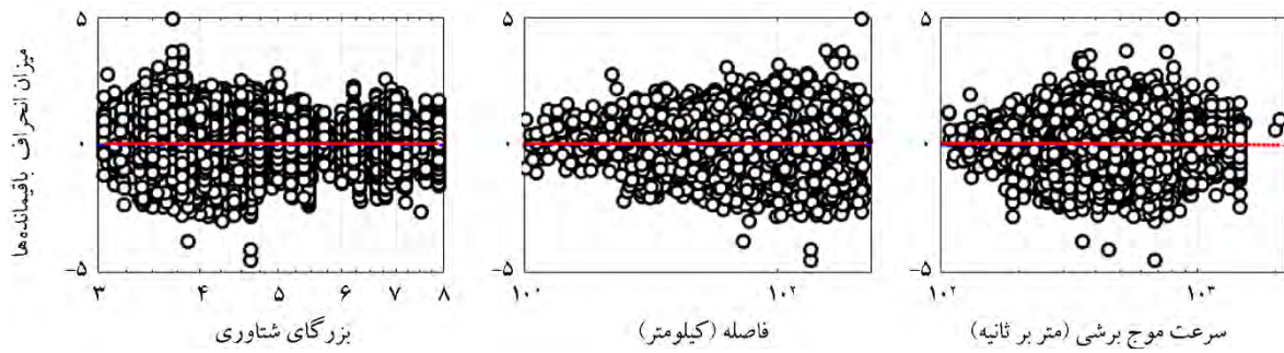
شکل (۲): توزیع باقیمانده‌های مدل CB 2014-GA برای پارامتر PGA (خط کامل، خط برازش داده شده بر روی باقیمانده‌ها در مقابل پارامترهای ورودی مختلف می‌باشد و خط چین، خط y=0 ، خط ایده‌آل برازش داده شده بر روی باقیمانده‌ها را نشان می‌دهد).
