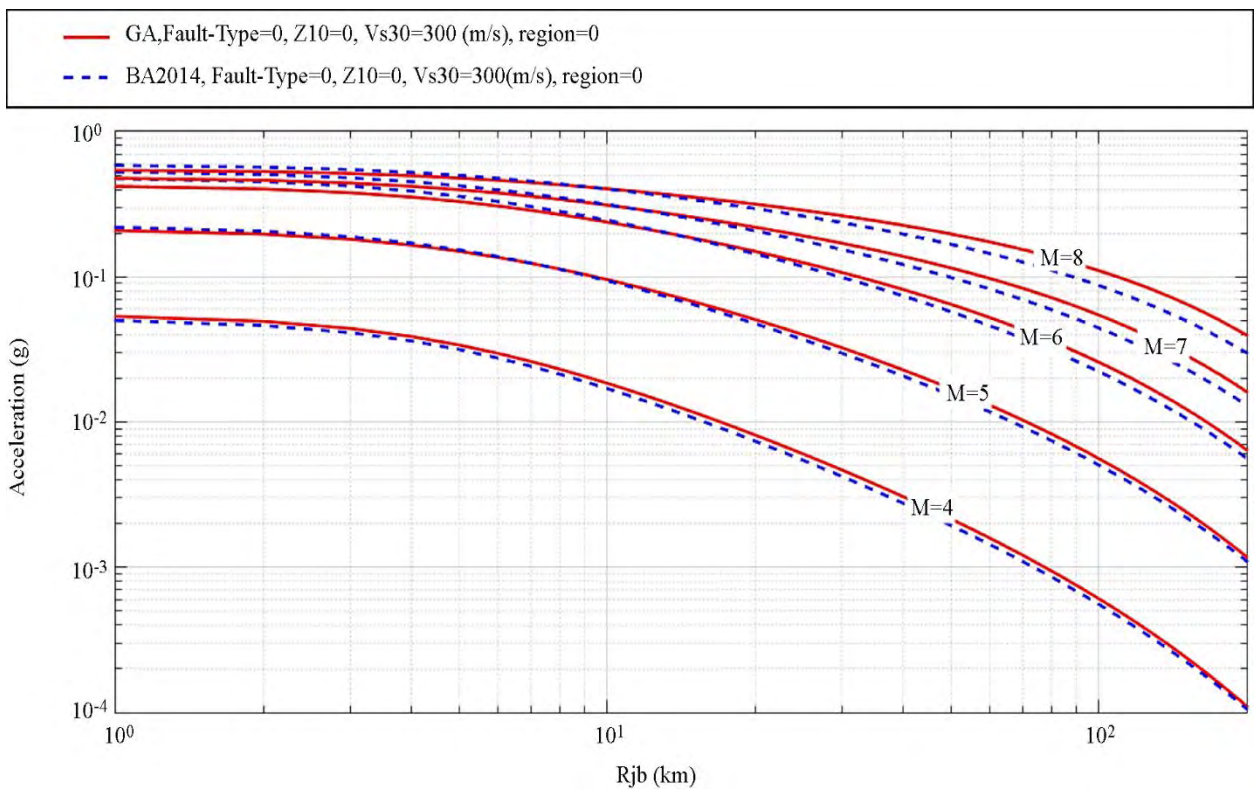
شکل (۱۵) مقایسه رابطه ارائه شده با رابطه BA 2014 در برابر پارامتر بزرگ (Fault-Type=0, Z10=0, Vs30=300(m/s), region=0).
