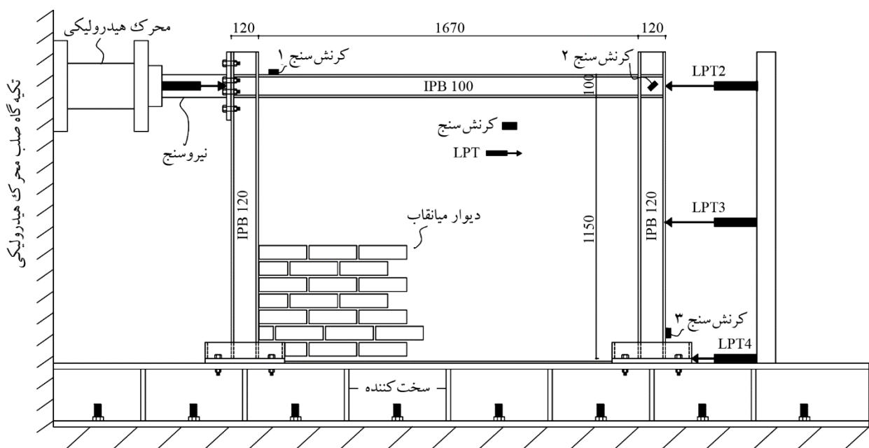
شکل (۱): پیکربندی آزمایش.
