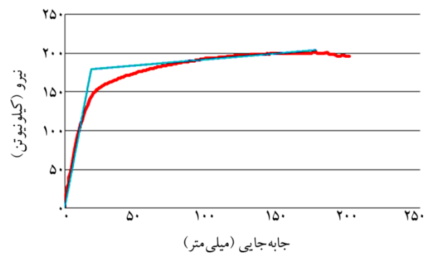
شکل (۳): نمودار نیرو - جاب‌جایی قاب F1.
