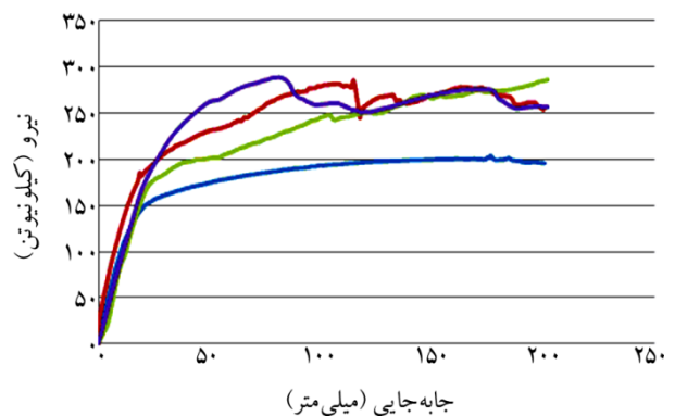
شکل (۱۰). نمودار نیرو - جابه‌جایی کل نمونه‌ها.
