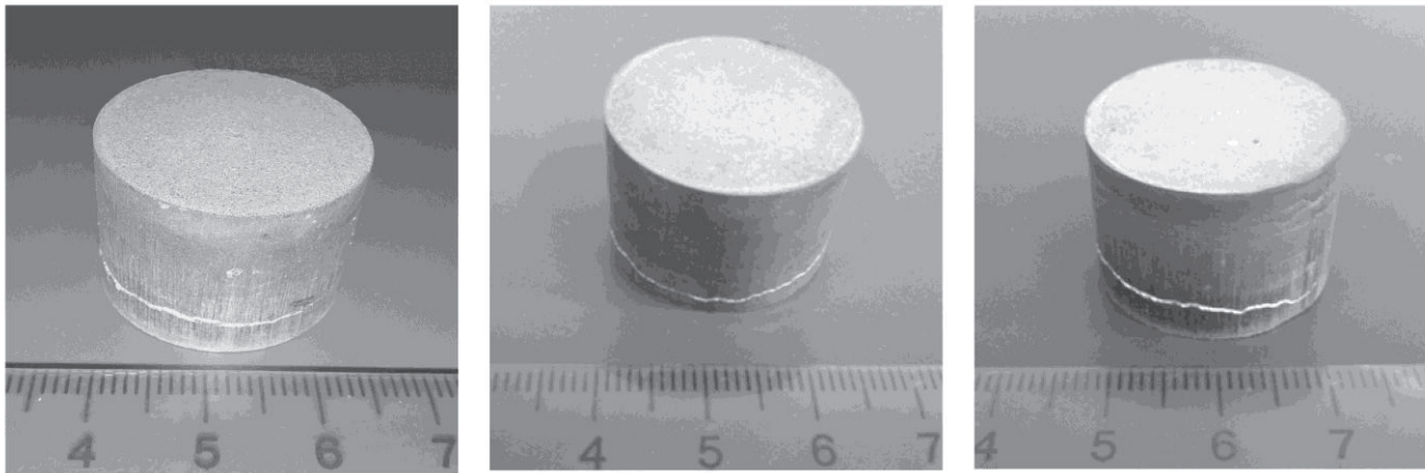
شکل ۷) نمونه های تابعی پنج لایه تف جوشی شده با اندازه ذرات SiC : (الف) ریز، (ب) متوسط و (ج) درشت.
