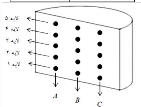
شکل ۸) شماتیک نمونه تابعی که در نواحی مختلف سختی سنجی شده.
