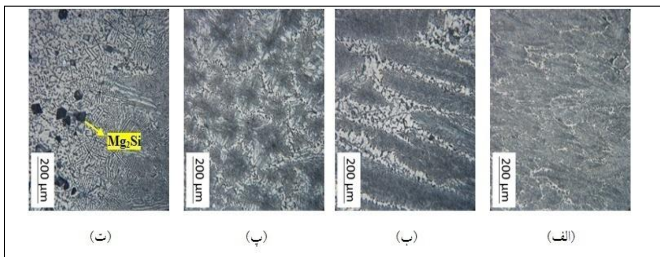
شکل ۲- ریزساختار میکروسکوپ نوری از مقاطع شعاعی مختلف استوانه ریخته شده از کامپوزیت \text{Al-13.8\%Mg}_2\text{Si} بدون بهساز (از الف) تا (ت) به ترتیب دلالت دارند بر ریزساختار خارجی ترین سطح استوانه تا داخلی ترین سطح آن [۱۳].
