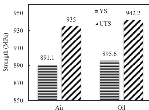
شکل (۸) تاثیر محیط سرمایش پس از آنیل بر استحکام آلیاژ Ti-6242.
