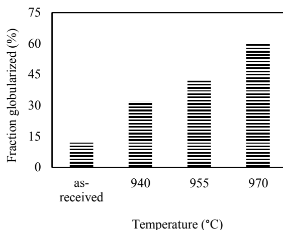
شکل (۴) تاثیر دمای آنیل بر کسر آلفای کروی.
