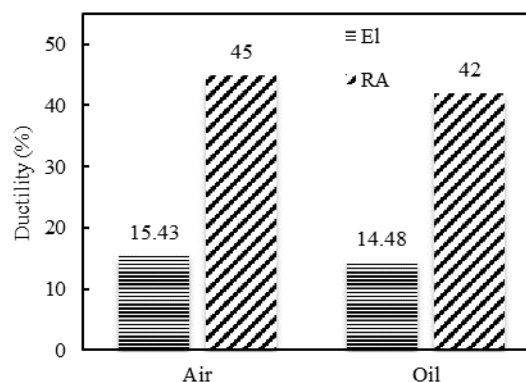
شکل (۹) تاثیر محیط سرمایش پس از آنیل بر داکتیلیته آلیاژ Ti-6242.
