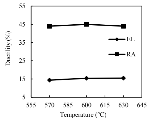
شکل (۱۲) تاثیر دمای پیرسازی بر داکتیلیته Ti-6242
