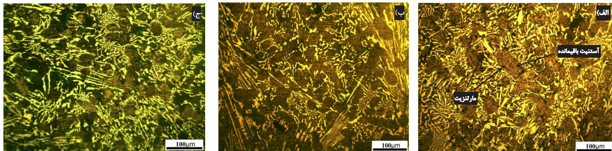
شکل ۴- تصاویر میکروسکوپ نوری پس از عملیات حرارتی با مقادیر مختلف آستنیت باقیمانده: الف) ۴۸٪ (نمونه ۱۶) ب) ۳۳٪ (نمونه ۹) و ج) ۲۶٪ (نمونه ۵).
