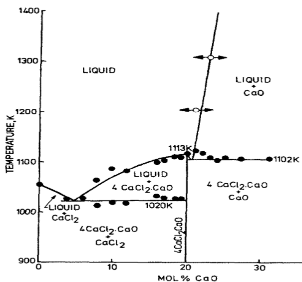
شکل ۲: دیاگرام فازی دوتایی [17] CaO-CaCl 2 .
