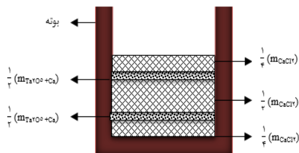
شکل ۱: شکل نمادین نحوه شارژ مواد اولیه در بوته
