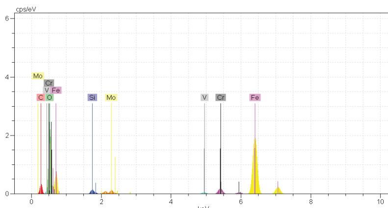
شکل ۶. الگوی حاصل از آنالیز عنصری آزمون EDS از نقطه B.
