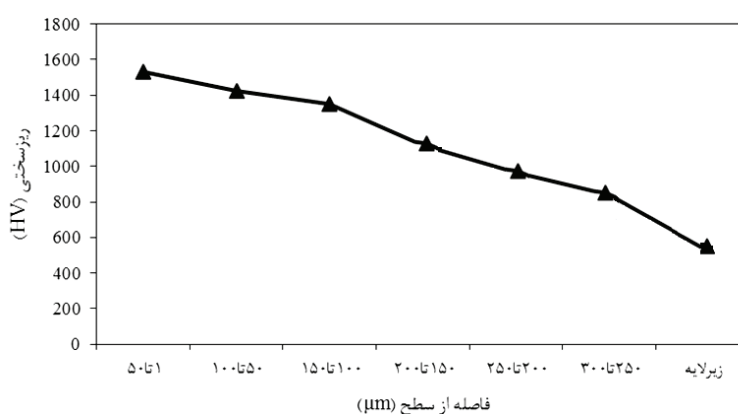
شکل ۳. پروفیل سختی منطقه کامپوزیت شده
