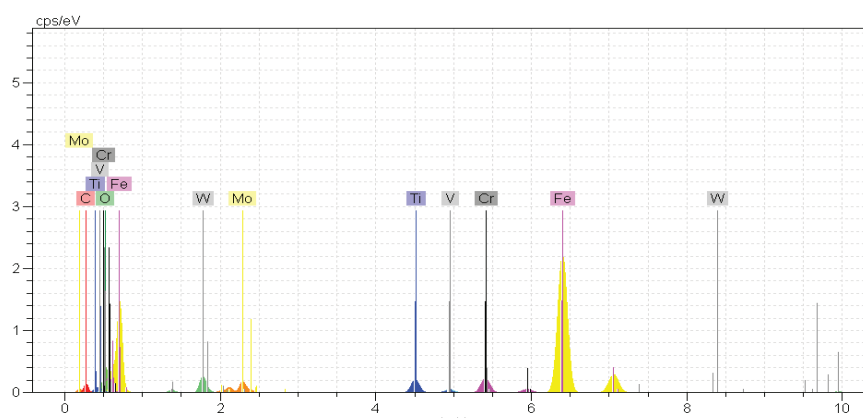
شکل ۹. الگوی حاصل از آنالیز عنصری آزمون EDS از نقطه B.
