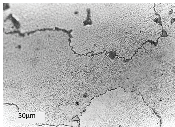
شکل ۵. تصویر میکروسکوپ نوری از مرفولوژی مرزدانه‌ها در سوپرآلیاژ IN738LC قبل از اعمال فرآیند فشار داغ
