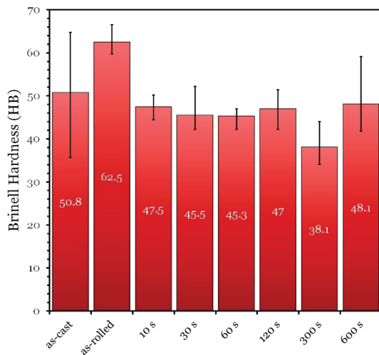
شکل ۹. تغییرات سختی برینل برای نمونه‌های مختلف.
