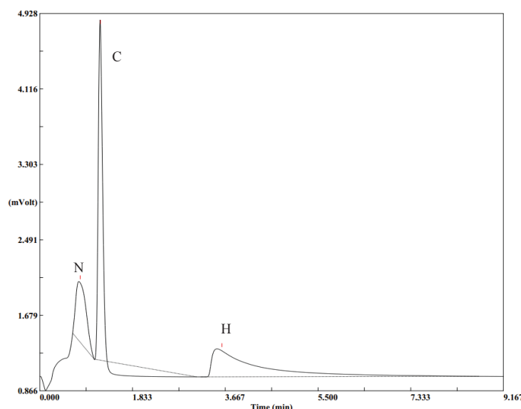
شکل ۶. منحنی کروماتوگرام آنالیز عنصری CHNS نانوذرات Fe 3 O 4 @TMOS.
