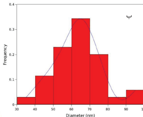
شکل ۲. تصویر SEM مربوط به (الف) نانوذرات Fe 3 O 4 و (ب) نانوذرات Fe 3 O 4 @TMOS در سمت چپ تصویر و نمودار توزیع اندازه آن‌ها در سمت راست.
