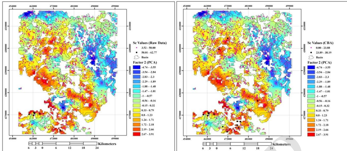
شکل ۸: نقشه‌های نقاط آنومالی (نقاط سیاه) و زمینه (نقاط صورتی) حاصل از روش CBA (سمت راست) و داده‌های خام (سمت چپ) مربوط به عنصر اسکاندیوم بر روی نقشه حاصل از کربجینگ معمولی مؤلفه دوم (PCA)
