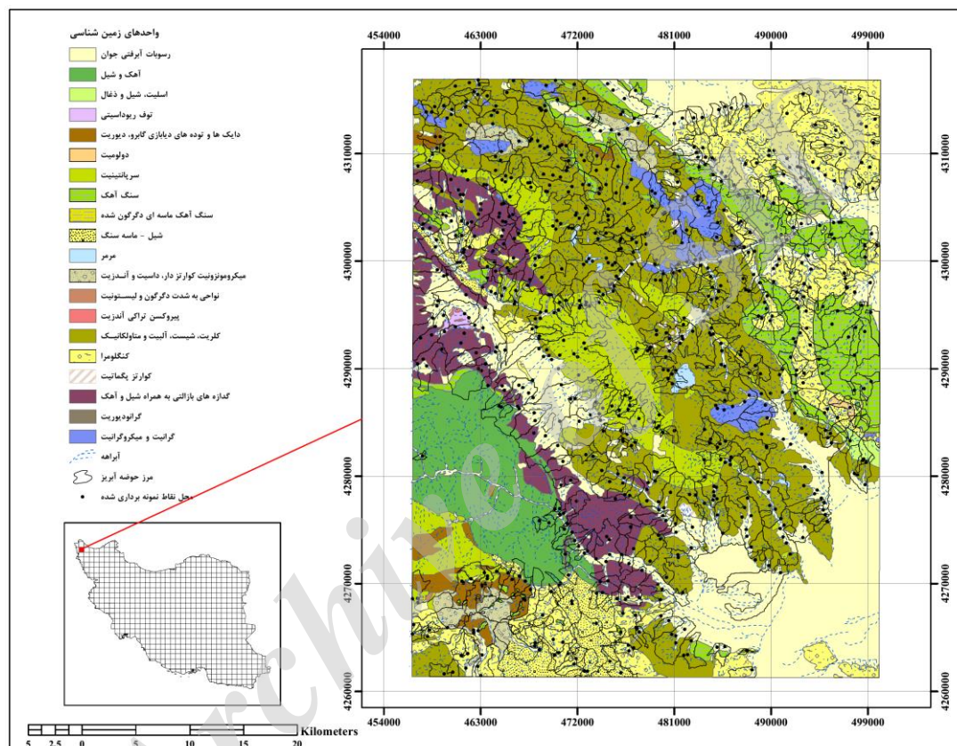
شکل ۱: موقعیت منطقه مورد مطالعه و نقشه زمین‌شناسی برگه خوی به همراه حوضه‌های آبریز منطقه (پاسیار و تراب، ۱۳۹۳، نقشه اصلی زمین‌شناسی توسط سازمان زمین‌شناسی کشور تهیه شده است)
