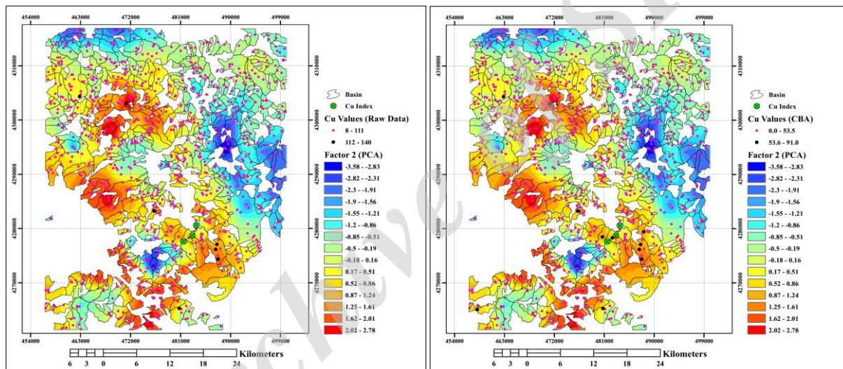
شکل ۹: نقشه‌های نقاط آنومالی (نقاط سیاه) و زمینه (نقاط صورتی) حاصل از روش CBA (سمت راست) و داده‌های خام (سمت چپ) مربوط به عنصر مس بر روی نقشه حاصل از کربجینگ معمولی مؤلفه دوم (PCA)
