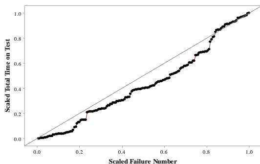
شکل ۴: آزمون ترسیمی روند سیستم لودر کاتریپلار
