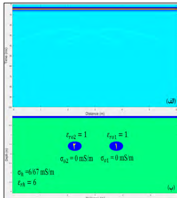
شکل ۸: الف) پاسخ GPR و ب) مدل هندسی - فیزیکی جفت استوانه افقی توخالی از جنس پلاستیک پی‌وی‌سی با قطر ۰/۵ متر واقع در عمق ۱/۲۵ متری. h: محیط میزبان و 0: شیء
