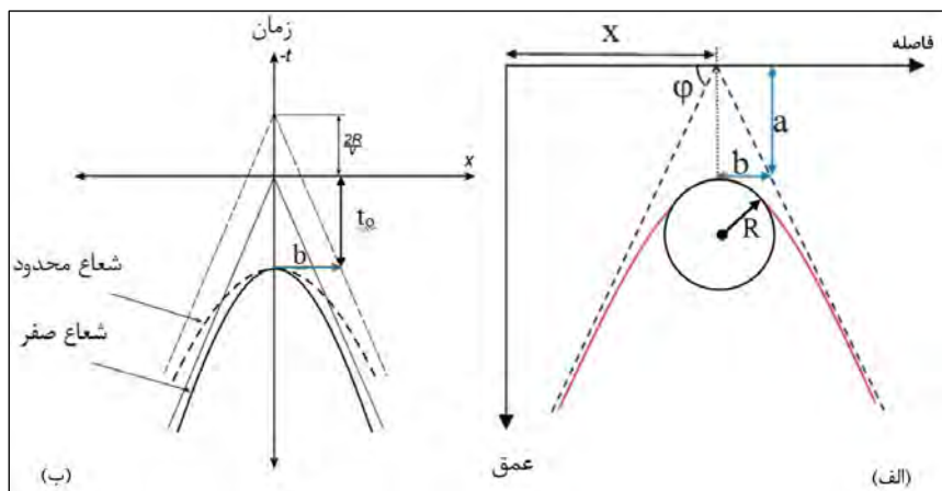
شکل ۲: الف) پاسخ نوعی GPR به صورت هذلولی برای یک هدف استوانه‌ای مدفون همراه با نمایش پارامترهای هندسی در حوزه مکانی؛ ب) پارامترهای مشخصه هذلولی در حوزه زمان- مکان (ویرایش شده از [۴])
