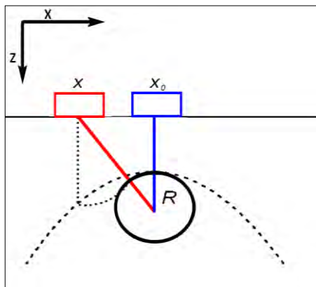
شکل ۳: نمایی از چگونگی روابط بین متغیرهای اصلی در بازتاب هذلولی.
