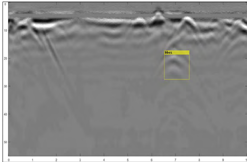
شکل ۱۵: آشکار شده شامل هذلولی بازتاب (پاسخ هدف) با استفاده از الگوریتم پیشنهادی ترکیبی با COD
