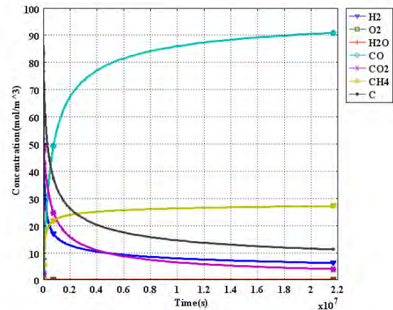
شکل ۵: نمودار غلظت گازهای تولیدی پس از اجرای اولیه مدل (در دمای 1273K و فشار 1MPa)
