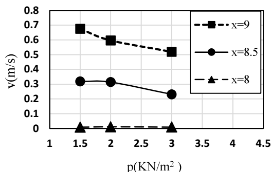
شکل (۱۷): نمایش رابطه سرعت جریان با فشار درون تیوپ: الف) Q=3.37 l/s، ب) Q=1.93 l/s
