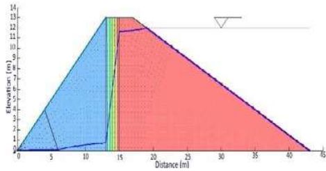
شکل (۱۵): نمایش خط فریاتیگ با نسبت k_c/k_a = 0.01
