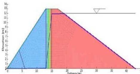
شکل (۱۶): نمایش خط فریاتیگ با نسبت k_c/k_a = 0.01
