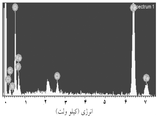
شکل ۴ طیف سنجی پراش انرژی پرتو ایکس؛ (۱) نانوذرات مغناطیسی و (۲) نانوذرات مغناطیسی درون گلیسرول مونولئات
