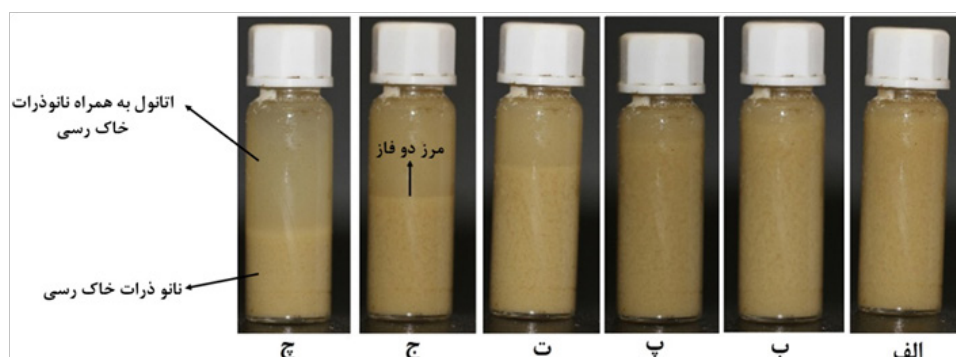
شکل ۴- پایداری نانوسیالات ۳٪ وزنی با سیال پایه اتانول بر حسب گذر زمان - الف: لحظه اولیه، ب: بعد از ۶ ساعت، ج: بعد از ۲۴ ساعت، ج: بعد از ۴۸ ساعت، ت: بعد از ۶ ساعت، ج: بعد از ۲۴ ساعت، ج: بعد از ۴۸ ساعت
