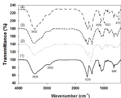
شکل ۵ طیف FTIR مربوط به هیدروژل کیتوزان (Cs) (۱)، Cs&Ph.ZnO@HAP (۲۵٪) (۲)، Cs&Ph.ZnO@HAP (۵٪) (۳) و Cs&Ph.ZnO@HAP (۱٪) (۴).
