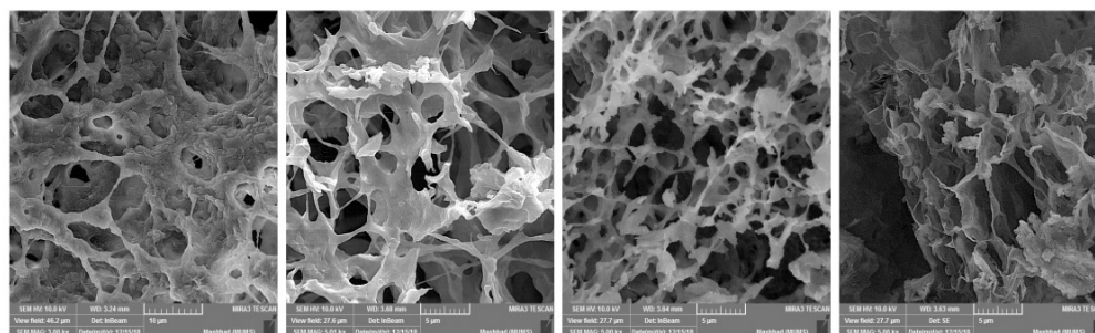
شکل ۶ تصاویر FESEM از هیدروژل کیتوزان (الف)، هیدروژل هیبریدی Cs&Ph.ZnO@HAP (۲۵٪) (ب) و Cs&Ph.ZnO@HAP (۵٪) (ج) و Cs&Ph.ZnO@HAP (۱٪) (د).
