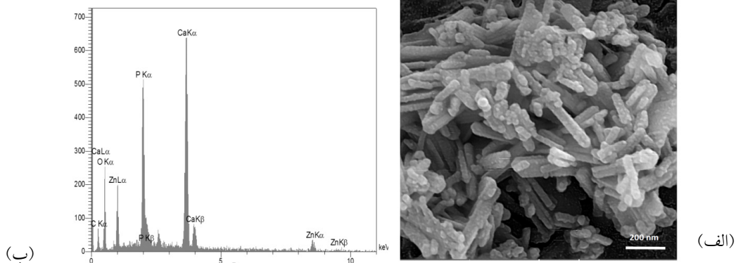
شکل ۲ تصویر FESEM نانوکامپوزیت Ph.ZnO@HAP (الف). طیف انرژی پرتو ایکس نانوکامپوزیت Ph.ZnO@HAP (ب).
