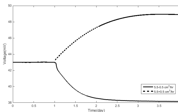
شکل ۳ نمودار تغییرات ولتاژ پیل سوختی میکروبی با تغییر در دبی ورودی به اندازه ± ۰/۵ Figure 3 Diagram of microbial fuel cell voltage changes with input flowrate of ± 0.5%
