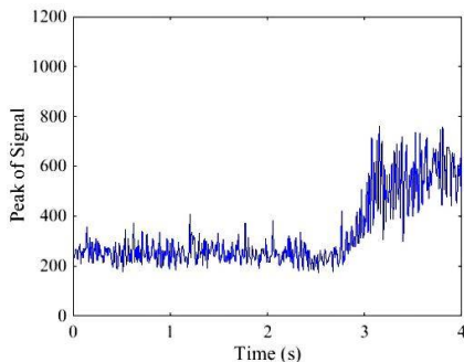
Fig. 9 The value of maximum peak of signal شکل 9 مقادیر حداکثر قله سیگنال شتاب
