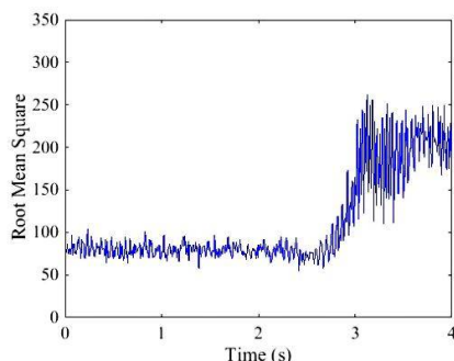
Fig. 8 The value of root mean square of signal شکل 8 مقادیر جذر میانگین مربعات سیگنال شتاب
