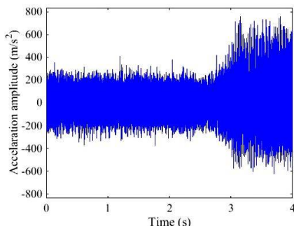
Fig. 6 Acceleration signal (sampling rate of 65536 Hz) شکل 6 سیگنال شتاب بر حسب زمان (نرخ نمونه برداری 65536 هرتز)
