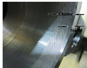
Fig. 5 The surface of workpiece test in table 5 شکل 5 سطح مقطع قطعه کار در آزمون جدول 5
