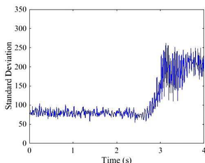
Fig. 7 The value of standard deviation of signal شکل 7 مقادیر انحراف معیار سیگنال شتاب
