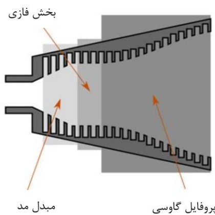
شکل ۴: طرح کلی هورن طراحی شده
